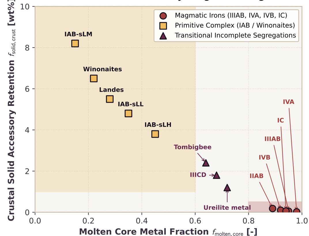
(d) Meteorite Parent Body Diagnostic Regimes
