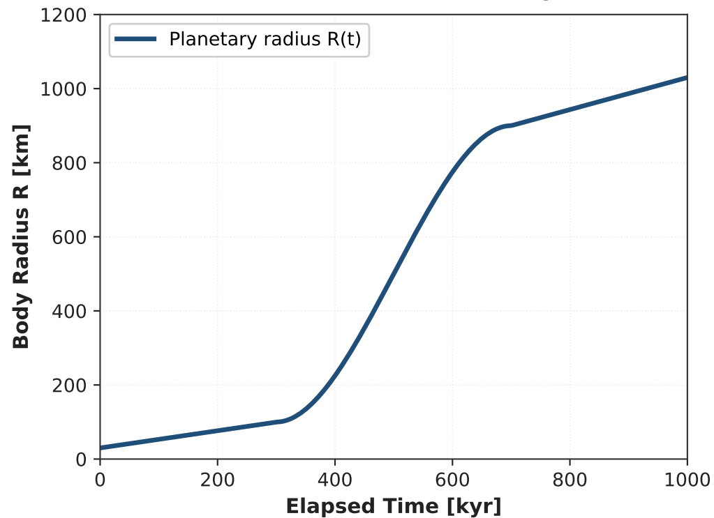
(d) Growth Evolution Across Regimes
