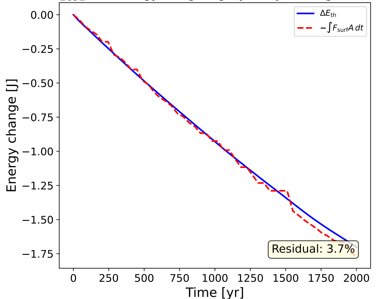
(d) Convective homogenization (no conduction)
