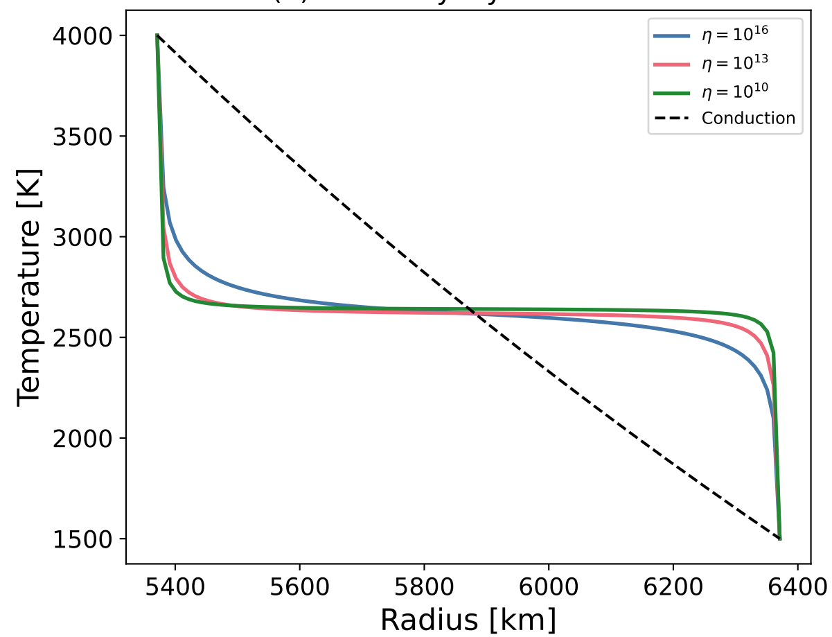
(d) Boundary layer structure
