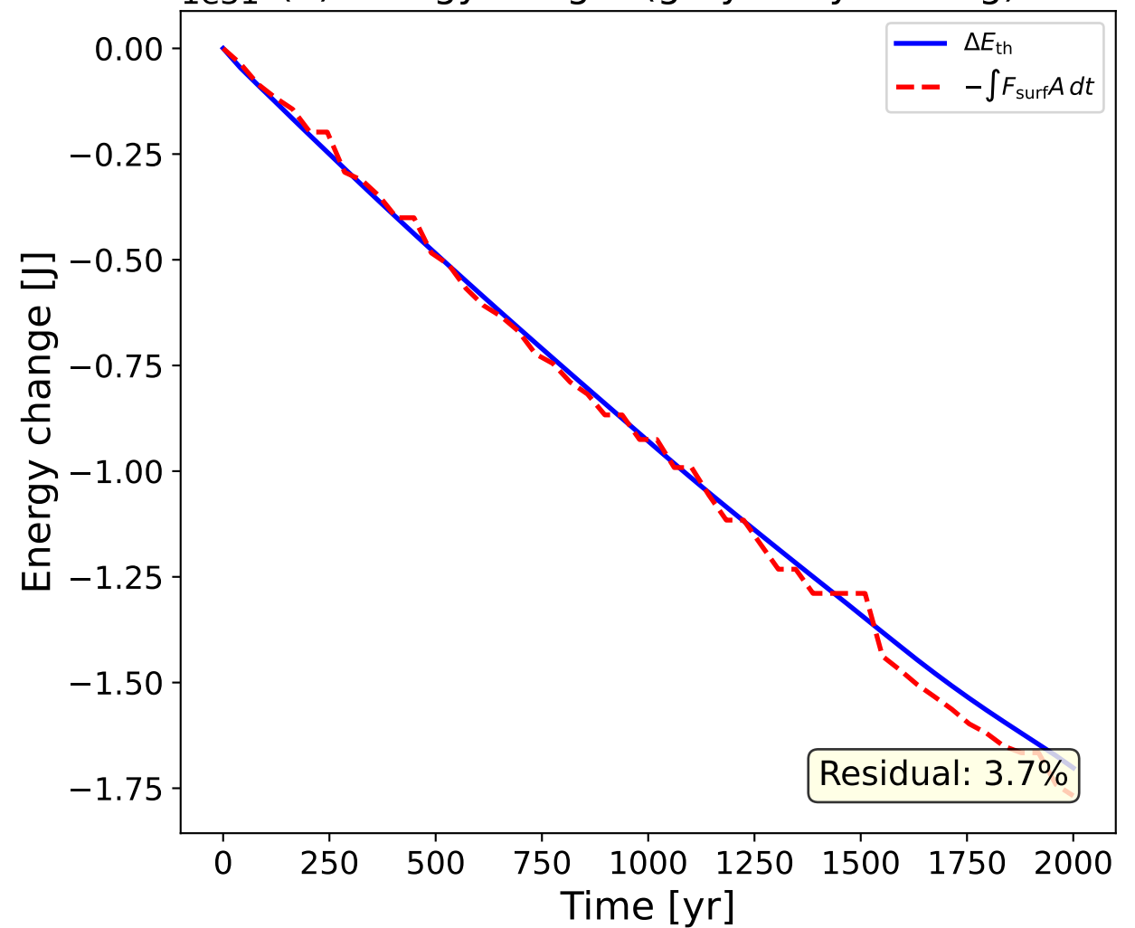
(d) Convective homogenization (no conduction)
