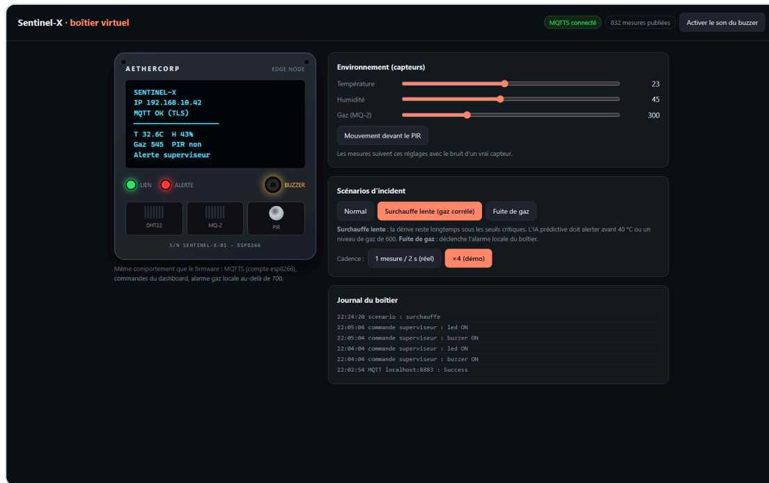
Boîtier virtuel pendant le scénario « surchauffe lente » : écran OLED, LEDs, buzzer, réglage des capteurs.
