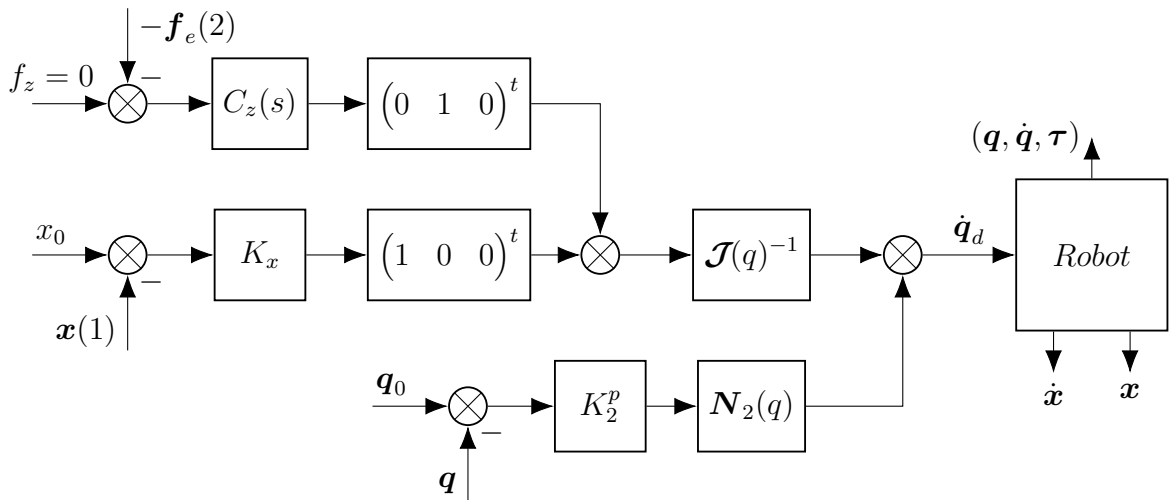
FIGURE 5 – Schéma bloc de la boucle de contrôle en transparence pour une tâche guidée sur une trajectoire virtuelle d'une dimension, sur un axe vertical parallèle à z
