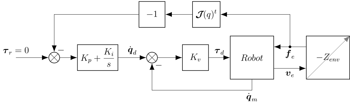
FIGURE 2 – Schéma bloc de contrôle en transparence avec capteur de force proposé par Lamy et al. (2009)
