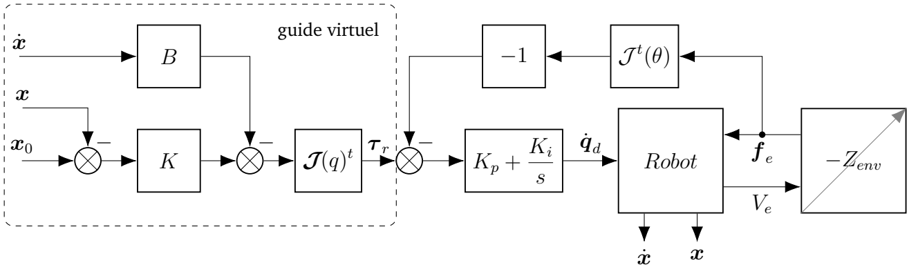
FIGURE 3 – Ajout d'un guide virtuel (Proportionnel Dérivé) à la boucle de transparence
