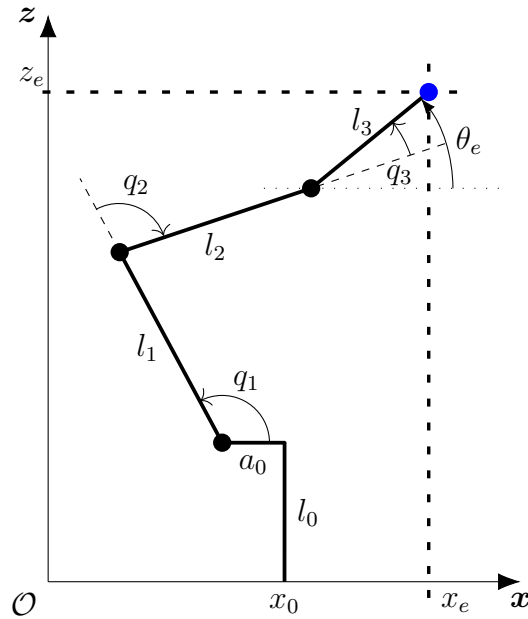
FIGURE 10 – Modèle simplifié du robot avec 3 articulations actionnées et 3 degrés de liberté
