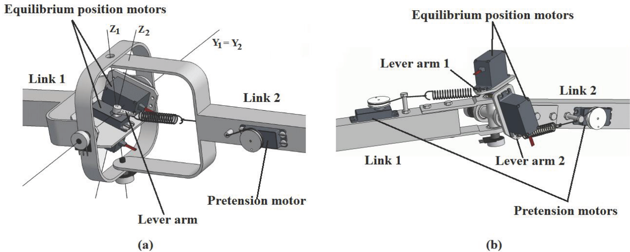
FIGURE 9 – MACCEPA à 2 DDL et 1 raideur variable (a) et MACCEPA complet avec 2 DDL et 2 raideurs variables indépendantes (b), (Weckx et al., 2014)
