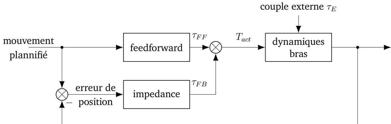
FIGURE 8 – Schéma bloc de contrôle en impédance avec utilisation de commande prédictive
