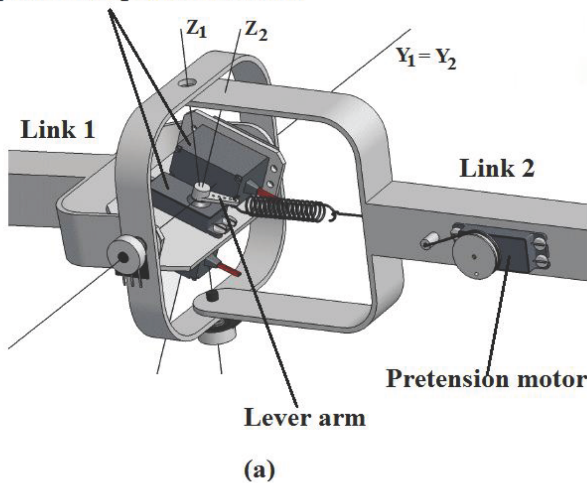
FIGURE 10 – MACCEPA à 2 DDL et 1 raideur variable (a) et MACCEPA complet avec 2 DDL et 2 raideurs variables indépendantes (b), (Weckx et al., 2014)
