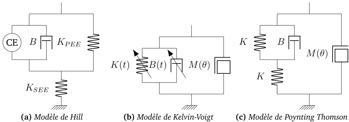
FIGURE 3 – Modèles mécaniques du bras humain
