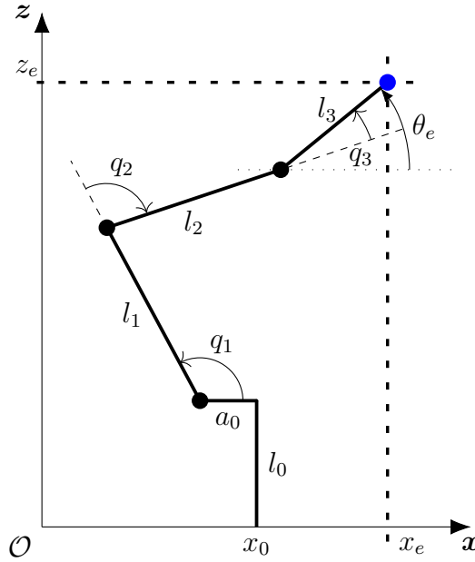
FIGURE 7 – Modèle simplifié du robot avec 3 articulations actionnées et 3 degrés de liberté
