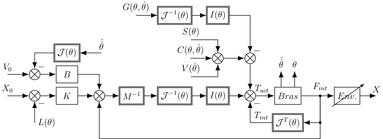
FIGURE 5 – Schéma équivalent décrivant la loi de commande (6) définie par Hogan (1985)
