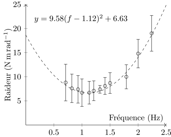
Figure 1.12: Reproduction des résultats obtenus par [Abe and Yamada, 2003], R^2 = 0.994
