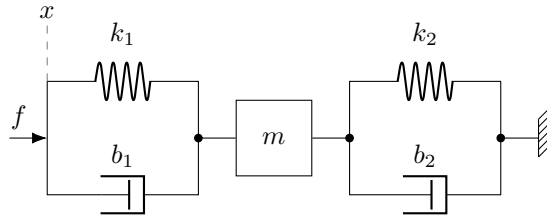
Figure 1.18: Modèle en impédance à 5 paramètres
