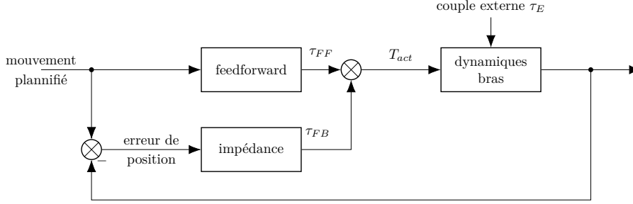
Figure 1.16: Schéma bloc de contrôle en impédance avec utilisation de commande prédictive, utilisé par [Tee et al., 2004]
