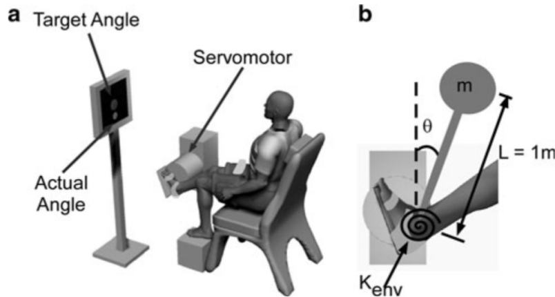
Figure 1.10: Banc expérimental pour une étude du contrôle de la cheville décrite par [Finley et al., 2012]. a) Les participants étaient assis, leur pied attaché à un servomoteur par l'interface d'une plaque rigide. b) Les participants contrôlaient une charge haptique instable qui se comportait comme un pendule inverse supporté par un ressort angulaire de raideur K_{env} . Le pendule simulé avait une masse équivalant à 25 % de la masse du participant et d'une hauteur de 1 m.
