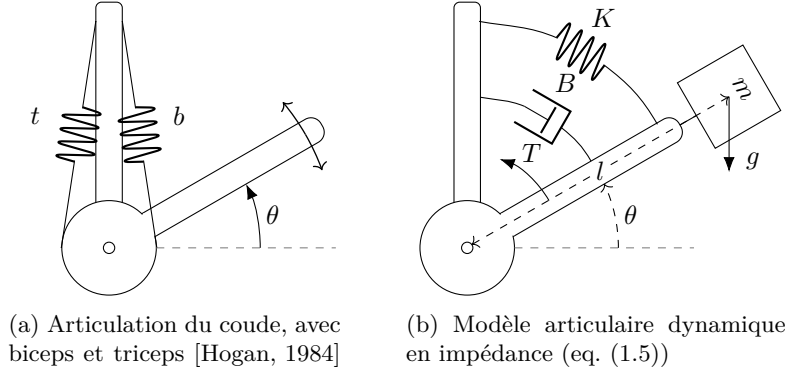
Figure 1.11: Modélisation simpliste de l'articulation du coude, avec l'action agoniste du biceps b et antagoniste du triceps t . Les muscles sont considérés comme de simple raideur variable, l'inertie du bras, la viscosité des muscles ainsi que le couple gravitationnel sont pris en compte lors des calculs présentés par [Hogan, 1984]. Ce modèle est valide pour de faibles vitesses (linéarisation de la viscosité), et de petites variations de posture (la dépendance articulaire [Rack and Westbury, 1969, Vredenburg and Rau, 1973] étant négligée).
