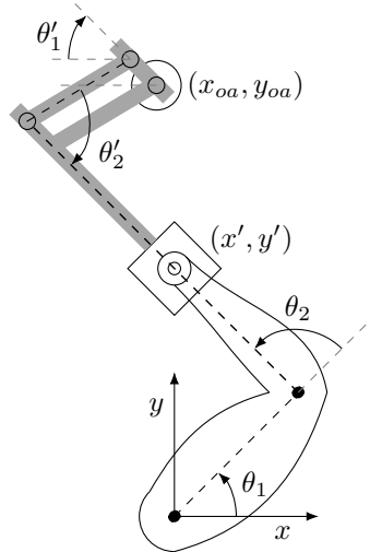
Figure 1.14: Expérience décrite par [Mussa-Ivaldi et al., 1985], avec le manipulandum maintenue par sa poignée (x', y') dans différentes postures. Vue de haut avec le centre du repère fixé sur l'articulation de l'épaule.
