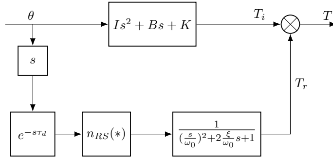
Figure 1.13: Modèle des propriétés intrinsèques de la cheville, avec la contribution des réflexes représentée par un modèle de Hammerstein, avec la non linéarité statique n_{RS} .
