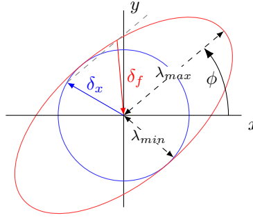
Figure 1.15: Exemple d'ellipse avec un déplacement \delta_x (bleu) sur le cercle unitaire, et la force de restitution (rouge) non-colinéaire induite, que l'on obtient grâce à l'intersection de la droite parallèle à l'axe principal passant par \delta_x et l'ellipse.
