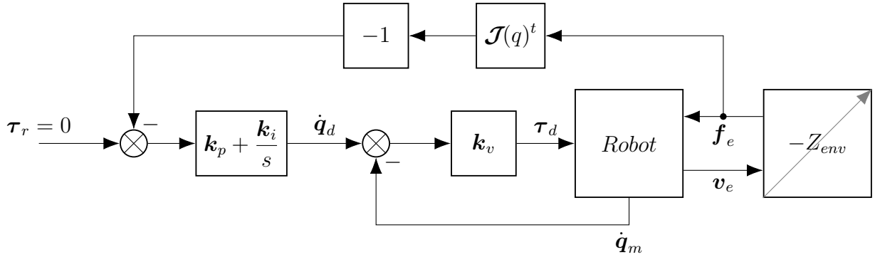
FIGURE 3 – Schéma bloc de contrôle en transparence avec capteur de force proposé par Lamy et al. (2009)
