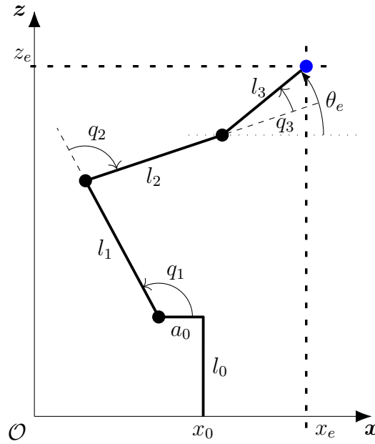
FIGURE 14 – Modèle simplifié du robot avec 3 articulations actionnées et 3 degrés de liberté
