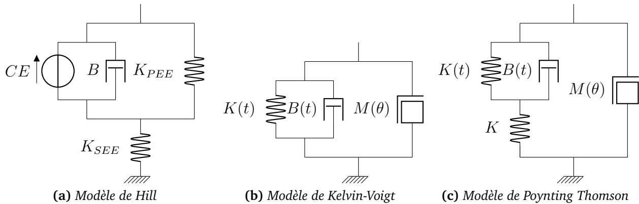
FIGURE 3 – Modèles mécaniques du bras humain
