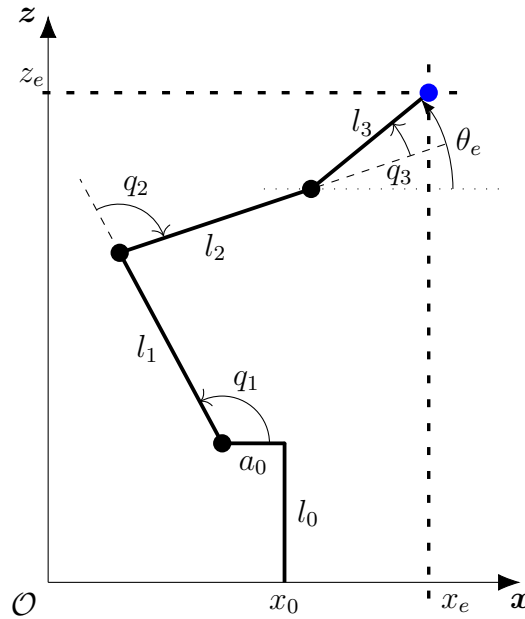
FIGURE 18 – Modèle simplifié du robot avec 3 articulations actionnées et 3 degrés de liberté
