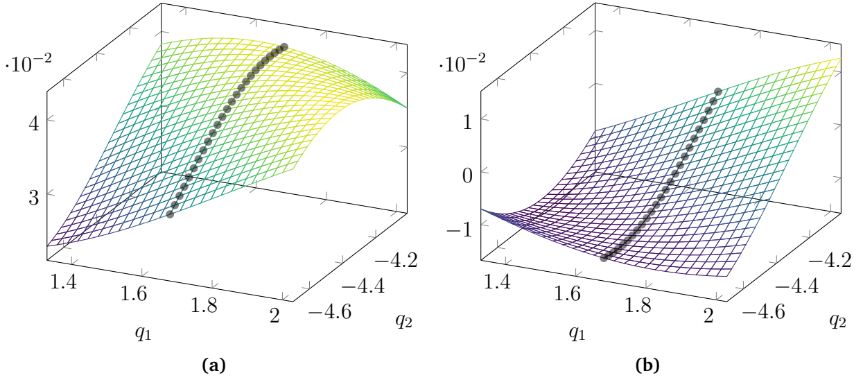
FIGURE 19 – Variations des termes matriciels de (E.2), pour q_3 = 1.5 . La position articulaire q_1 = 1.68 est signalée par des marqueurs circulaires. (a) Termes de la diagonale influençant la position en x , (a) termes de couplages en x qui sont multipliés par f_z . Les positions articulaires sont données en radians.
