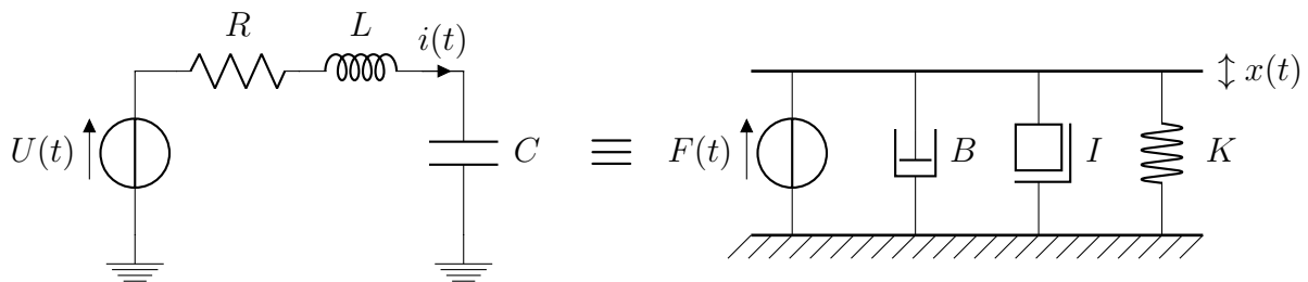
FIGURE 17 – Analogie électricité - mécanique
