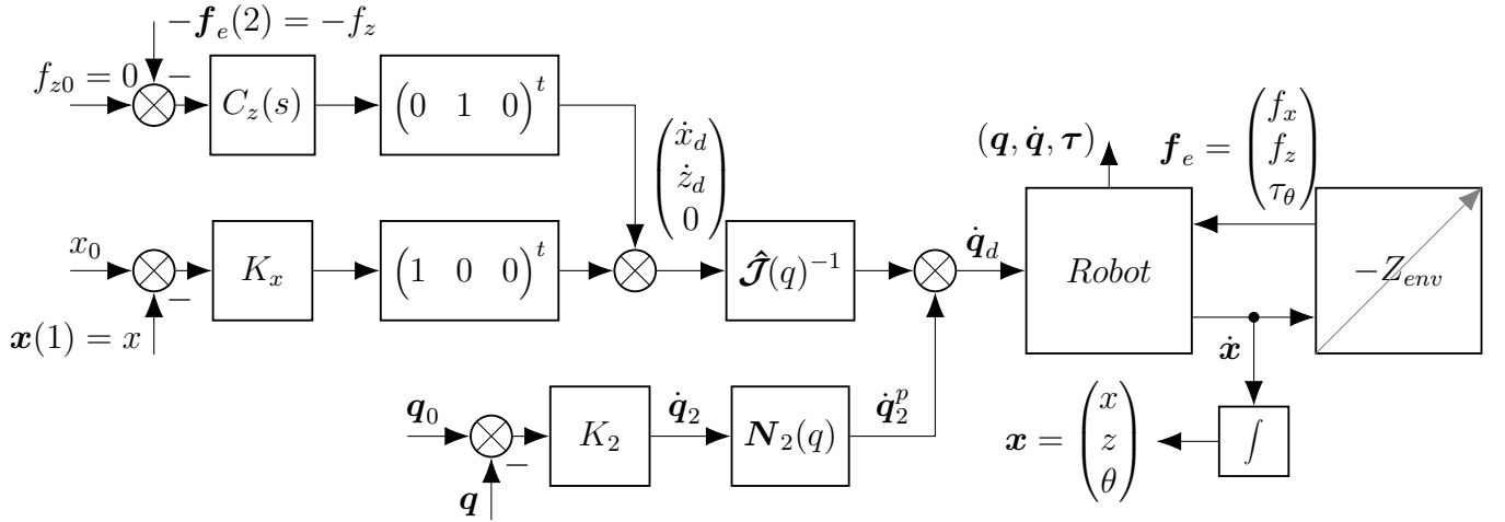
FIGURE 5 – Schéma bloc du contrôle interactif du robot, pour une tâche guidée sur une dimension le long de z . \mathbf{f}_e représente les forces d'interaction dans le référentielle de la base du robot, \mathbf{q} les positions articulaires, \boldsymbol{\tau} les couples articulaires et \mathbf{x} les coordonnées cartésiennes de l'effecteur du robot. C_z = K_p + \frac{K_i}{s} est un correcteur Proportionnel Intégral (PI) responsable de la commande en admittance interactive.
