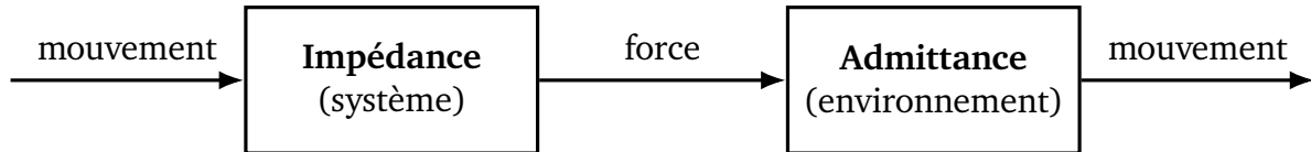
FIGURE 16 – Systèmes physiques : comme expliqué par Hogan (1985), l'environnement peut souvent être modélisé par une admittance, un système qui interagit avec, devra donc être considéré comme une impédance.
