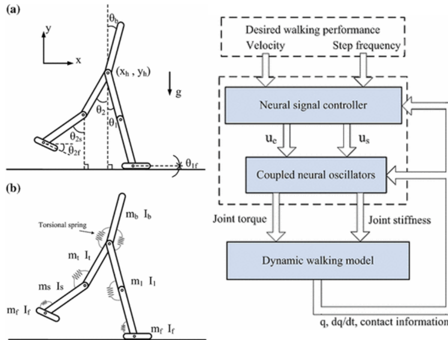
FIGURE 11 – A droite, le digramme décrivant le schéma de contrôle de ?, à gauche le modèle de bipède à 7 liens, (a) les degrés de liberté, (b) les ressorts de torsion.
