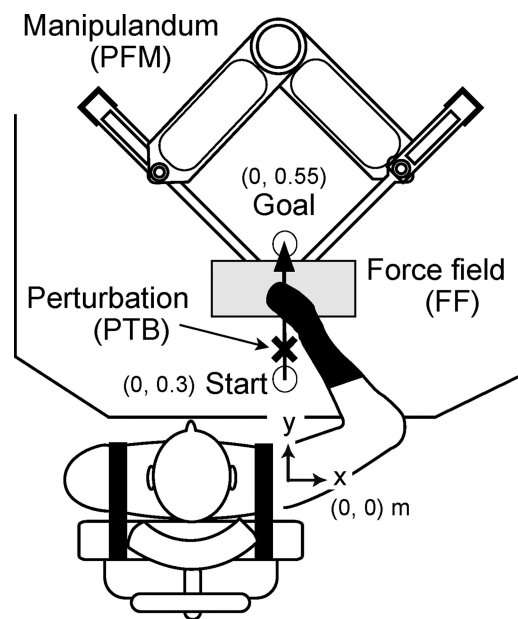
FIGURE 4 – Manipulandum utilisé par Kimura et al. (2006), proche de celui utilisé par les autres auteurs cités ci-après.
