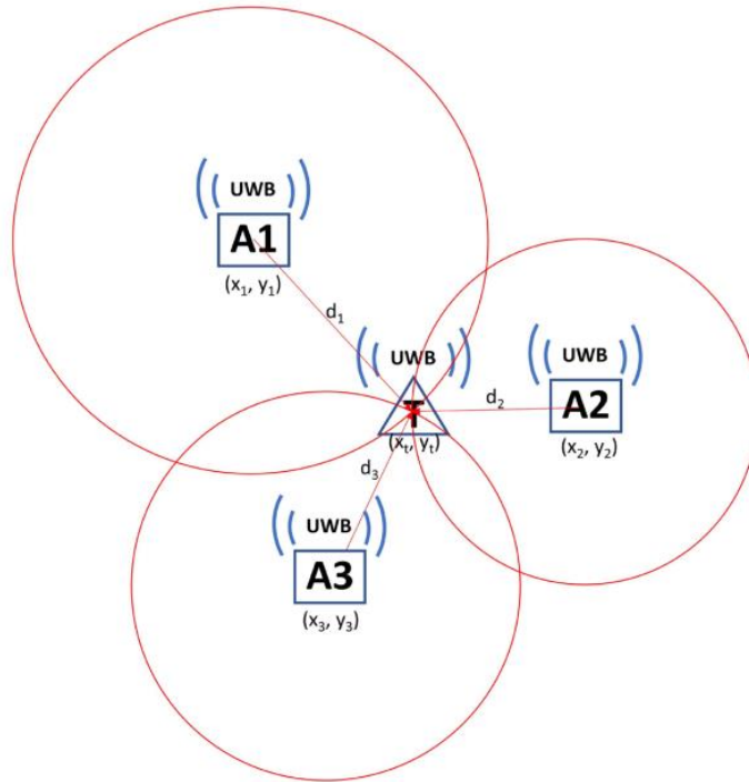
Рисунок 2.4 — Метод трилатерации
