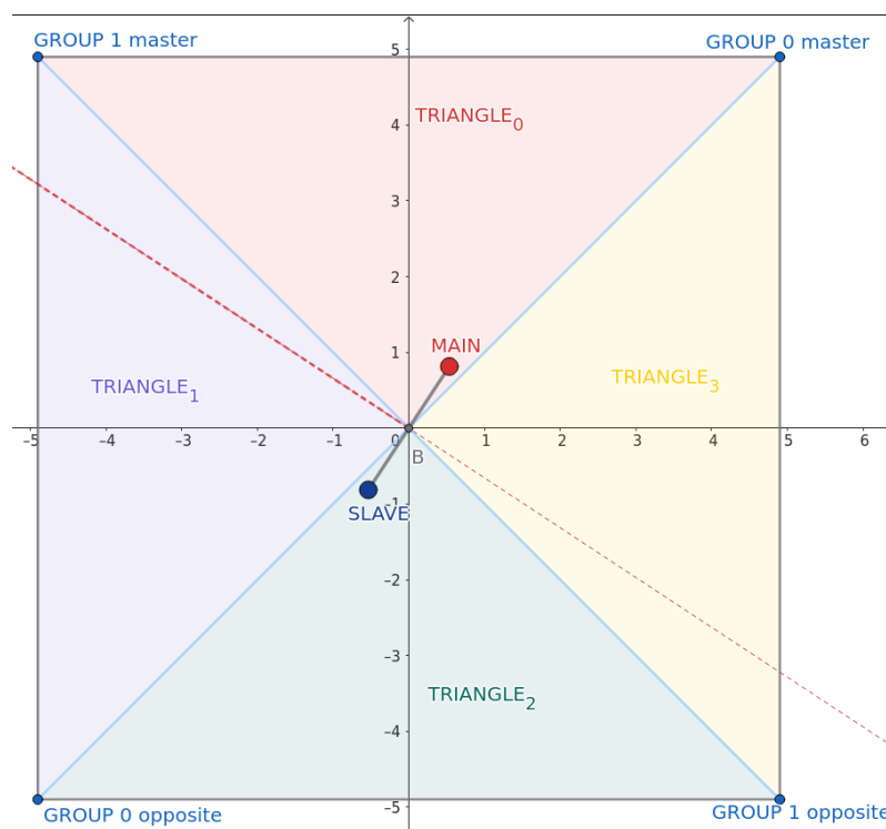
Рисунок 4.5 — Группы маяков на горизонтальной плоскости
