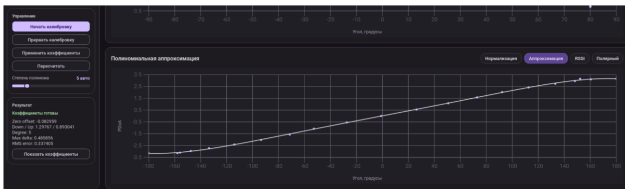
Рисунок 5.5 — Полиномиальная аппроксимация
