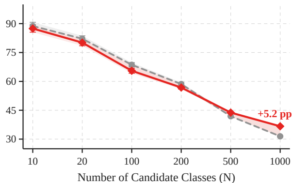
(f) Gemma-4-E4B
