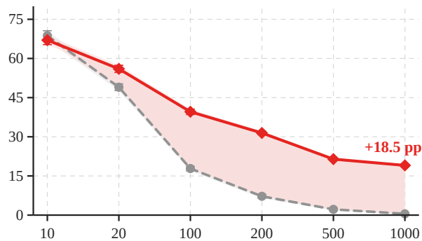
(d) DeepSeek-VL-7B-chat
