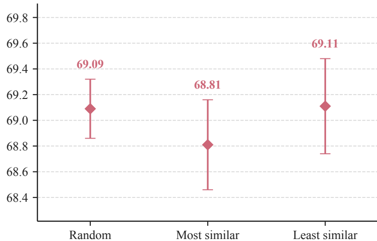
(b) Qwen3-VL-4B-Instruct
