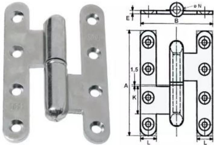
Paumelle acier zingué MONIN 110 x 60 Ø15,5, droite
