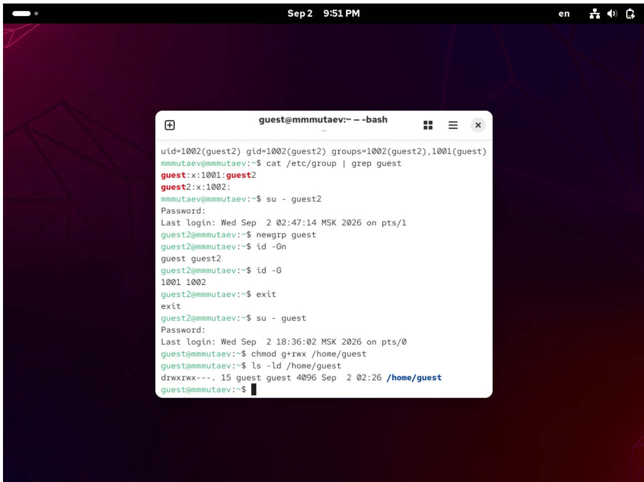
Рис. 3. Предоставление группе прав на /home/guest.
