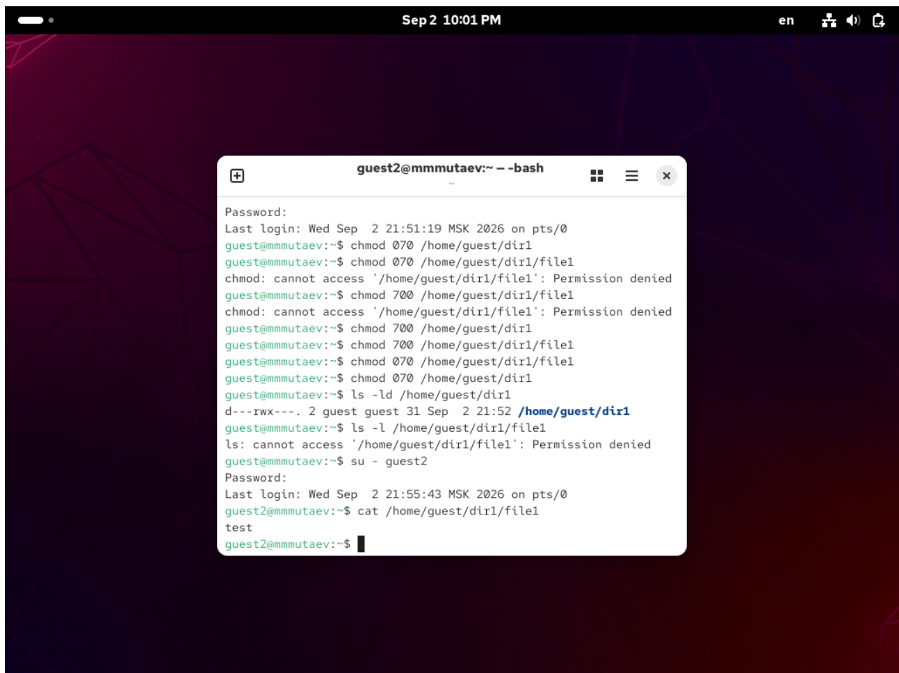
Рис. 6. Полные права для группы.
