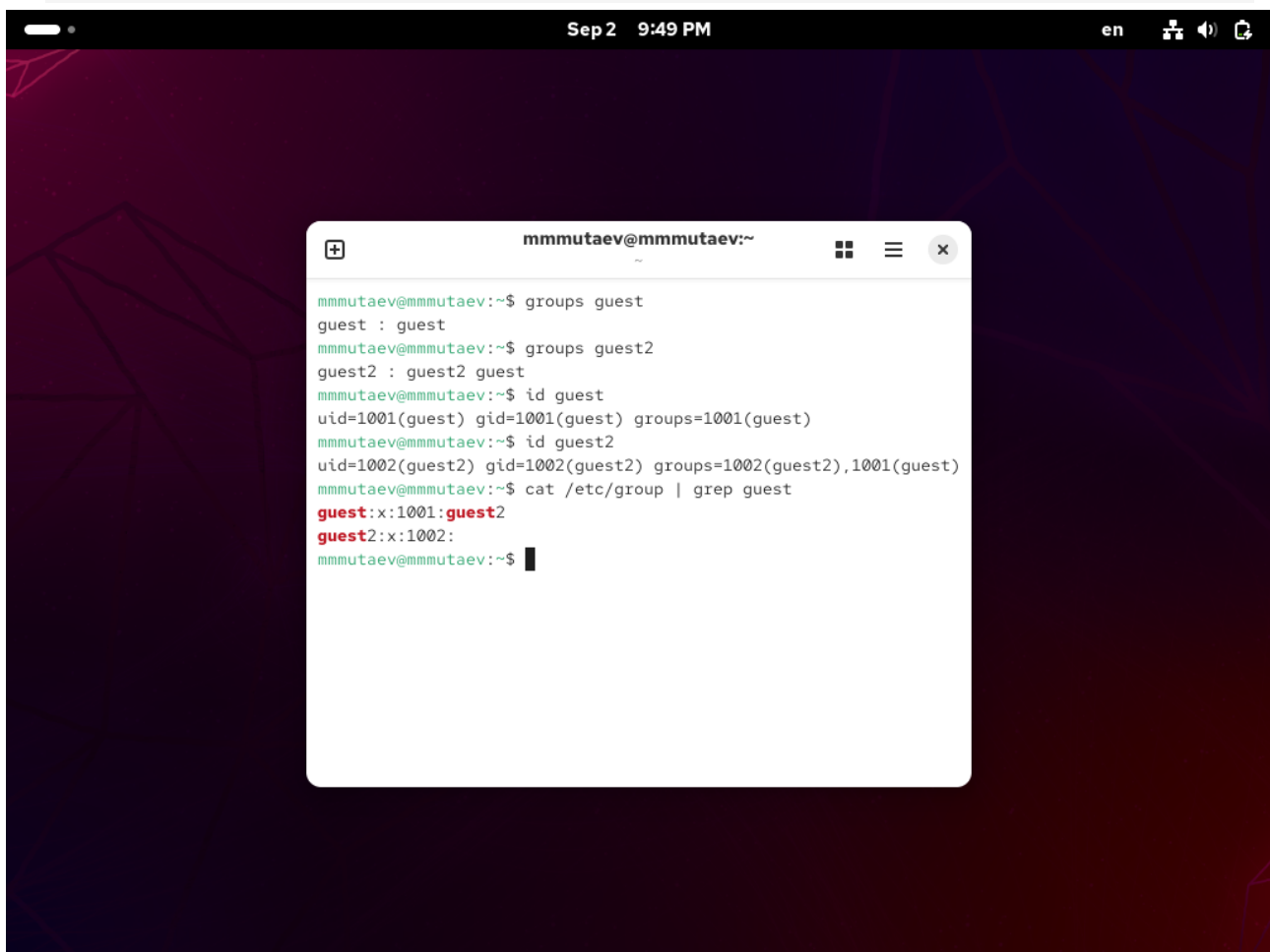
Рис. 1. Сведения о пользователях и группах.
