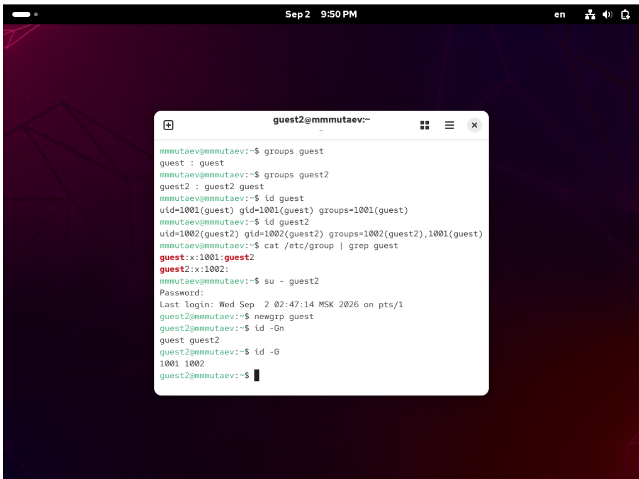
Рис. 2. Переход пользователя guest2 в группу guest.
