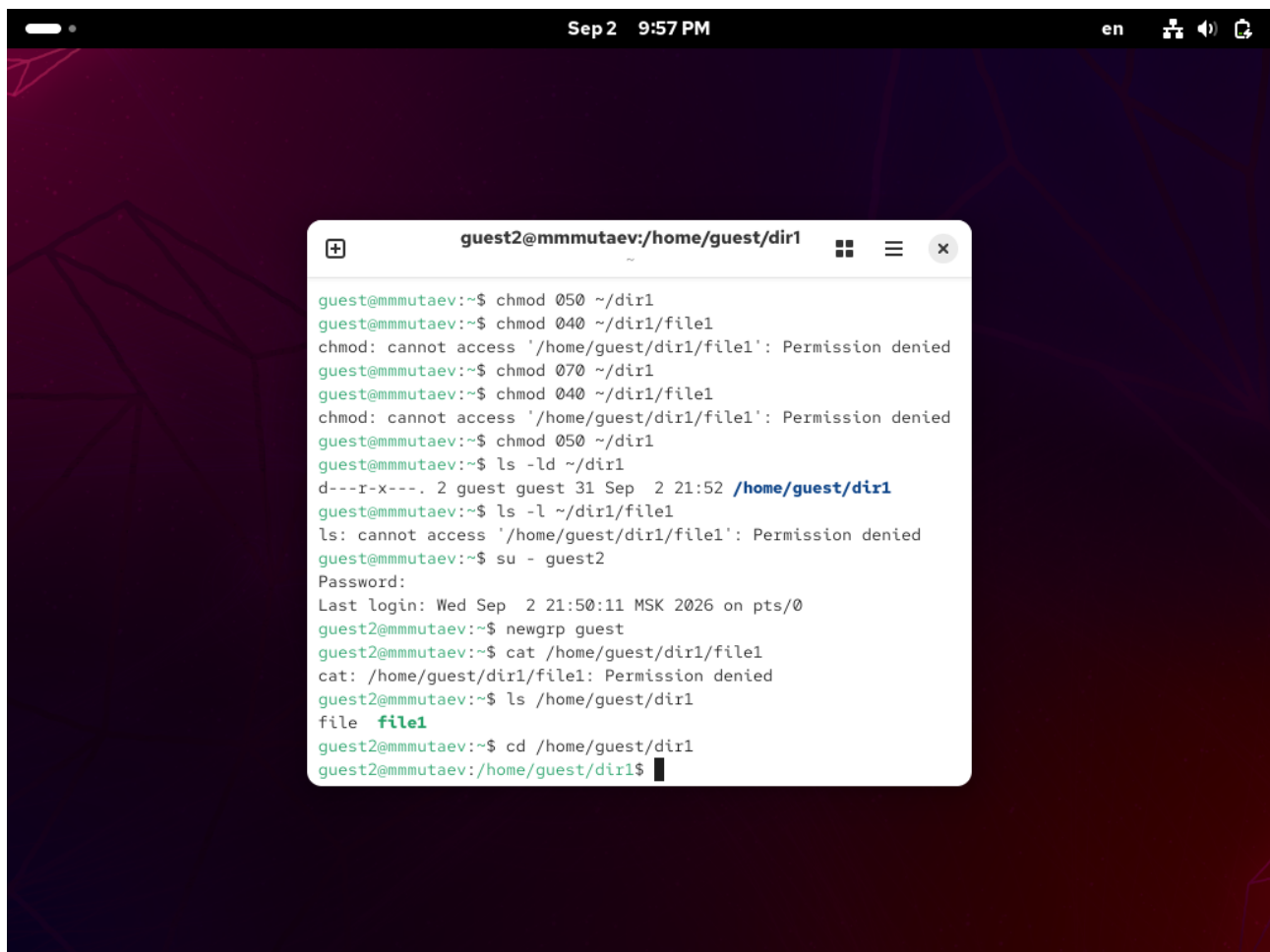
Рис. 5. Проверка прав от имени guest2.
