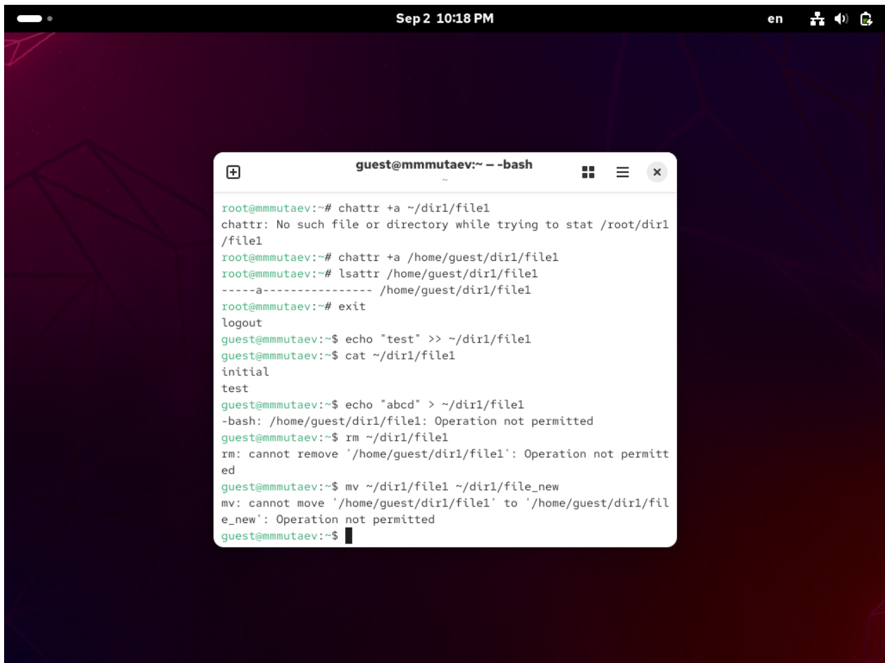
Рис. 5. Запрет удаления и переименования при атрибуте а.
