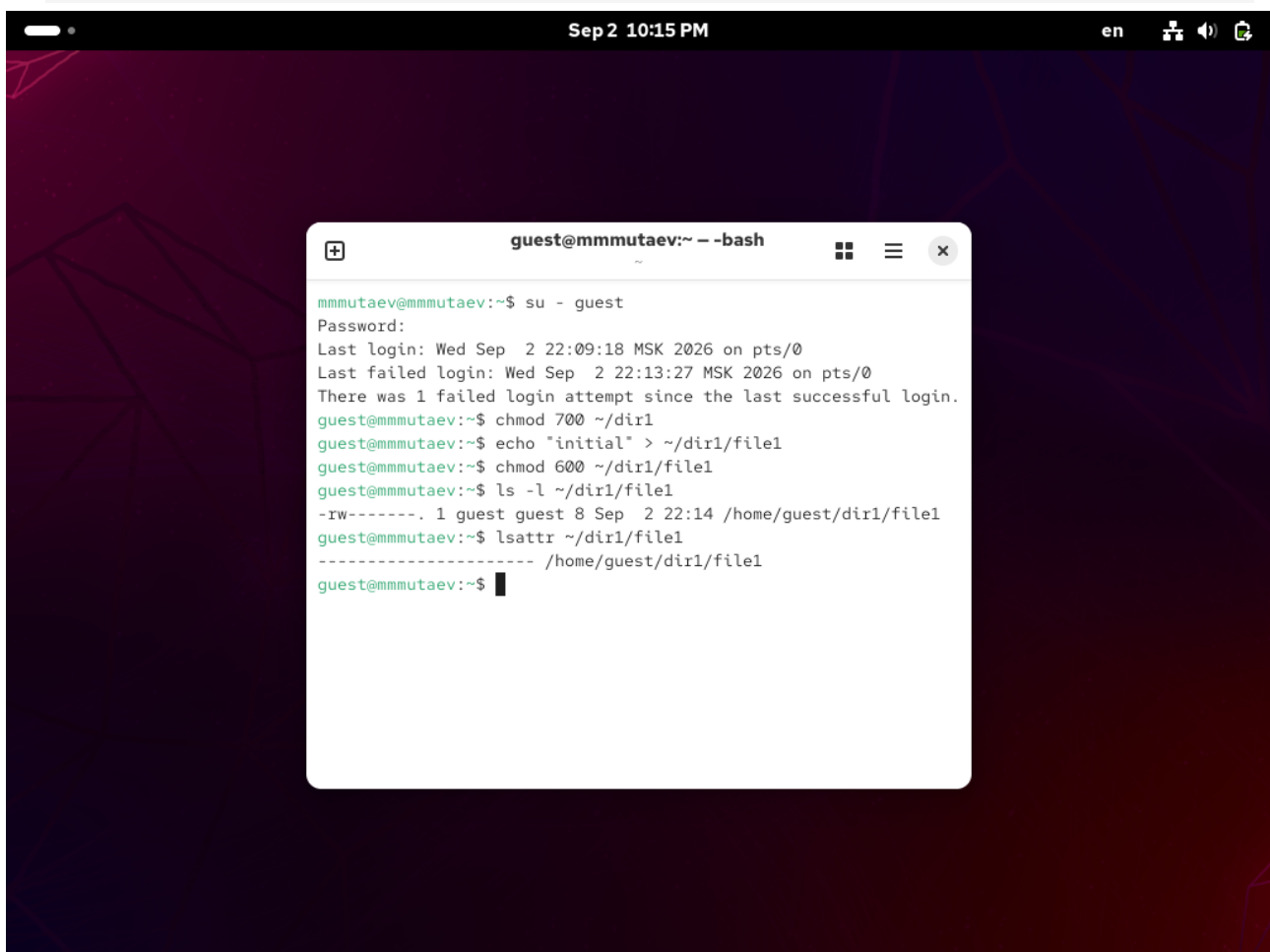
Рис. 1. Исходные права и расширенные атрибуты файла.
