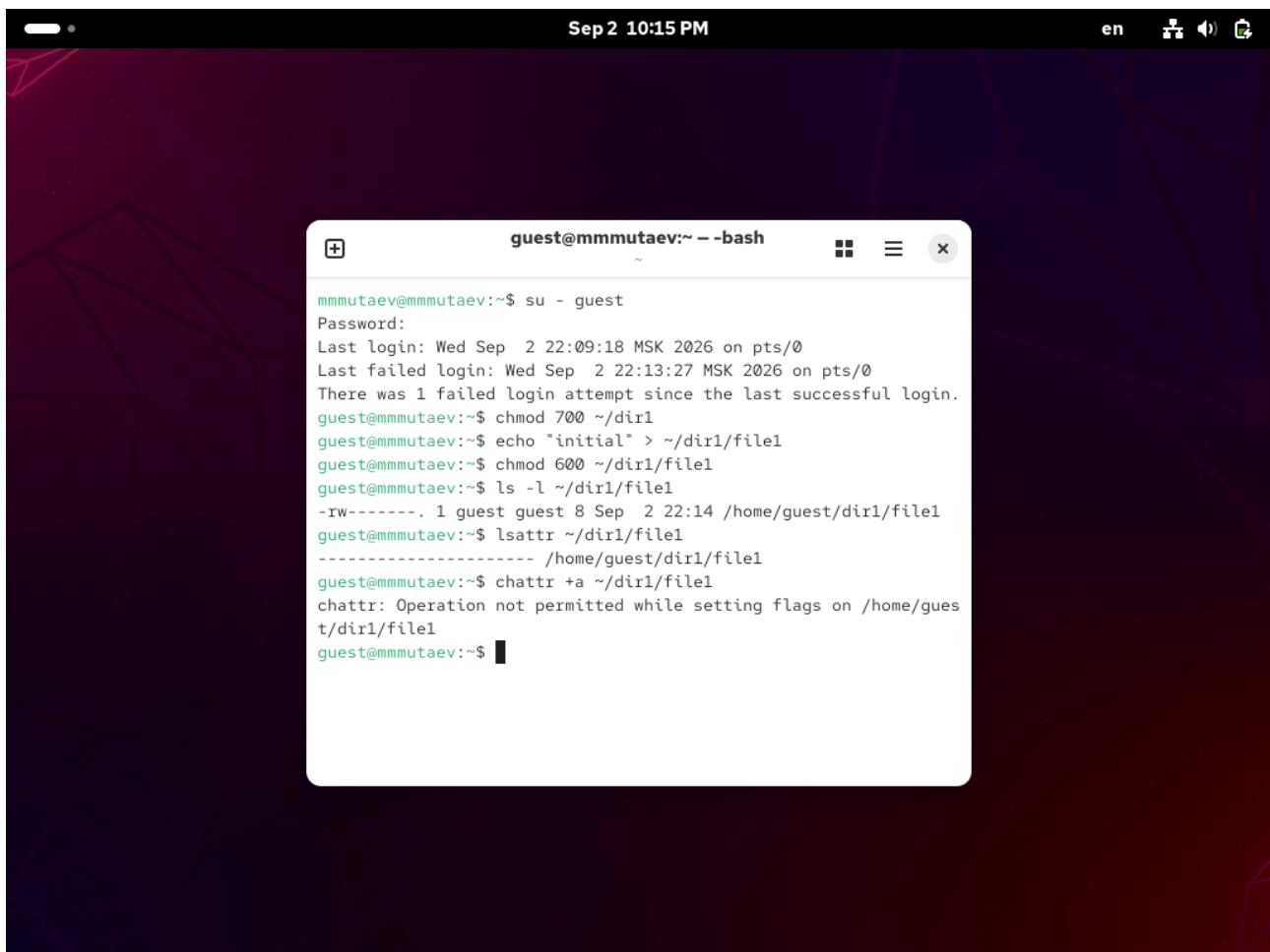
Рис. 2. Отказ при установке атрибута а обычным пользователем.
