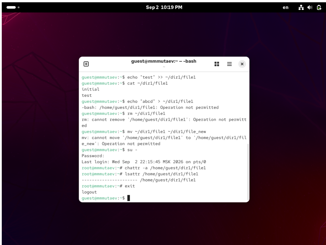
Рис. 6. Снятие атрибута a.
