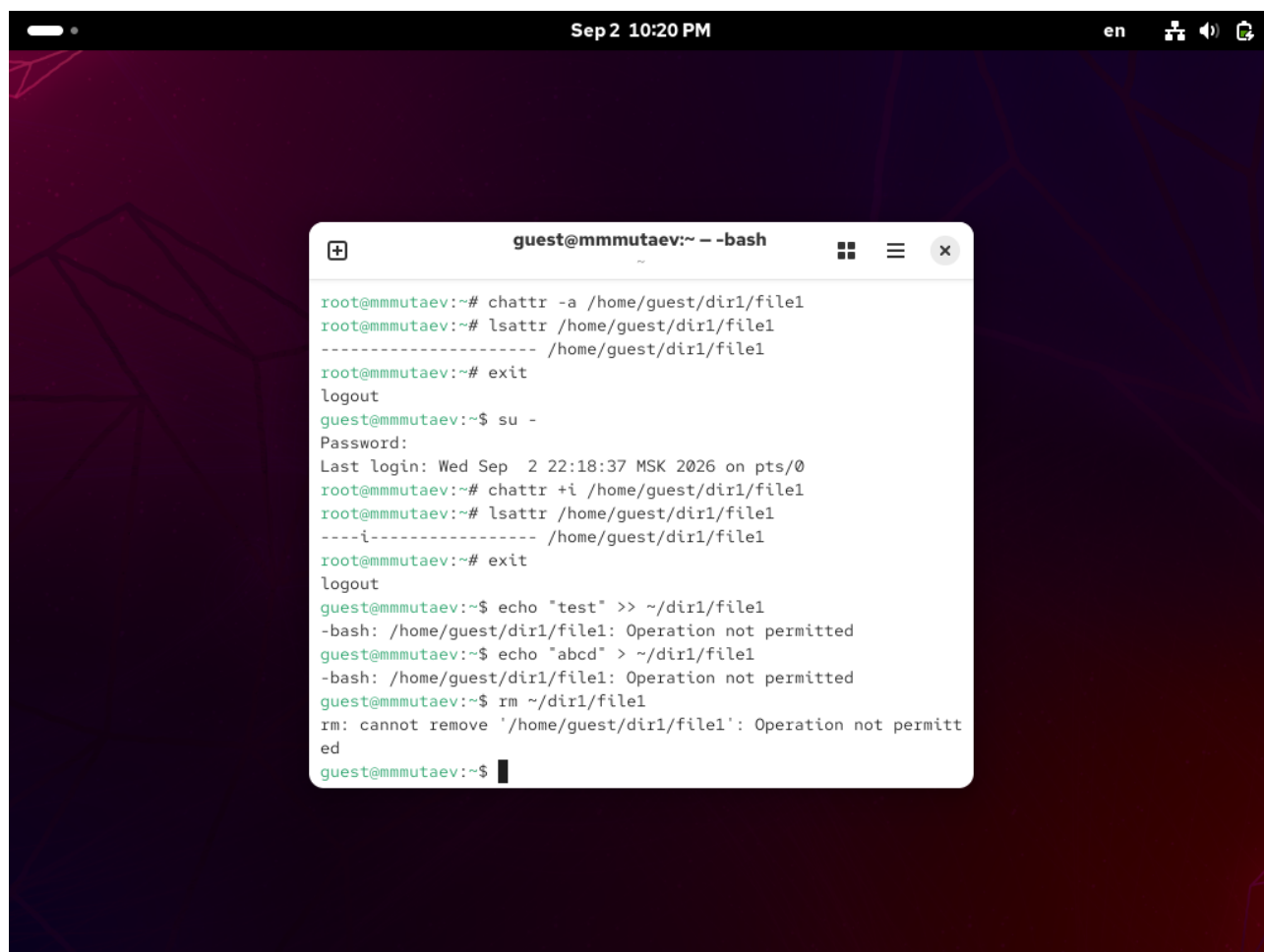
Рис. 8. Ограничения при атрибуте i.
