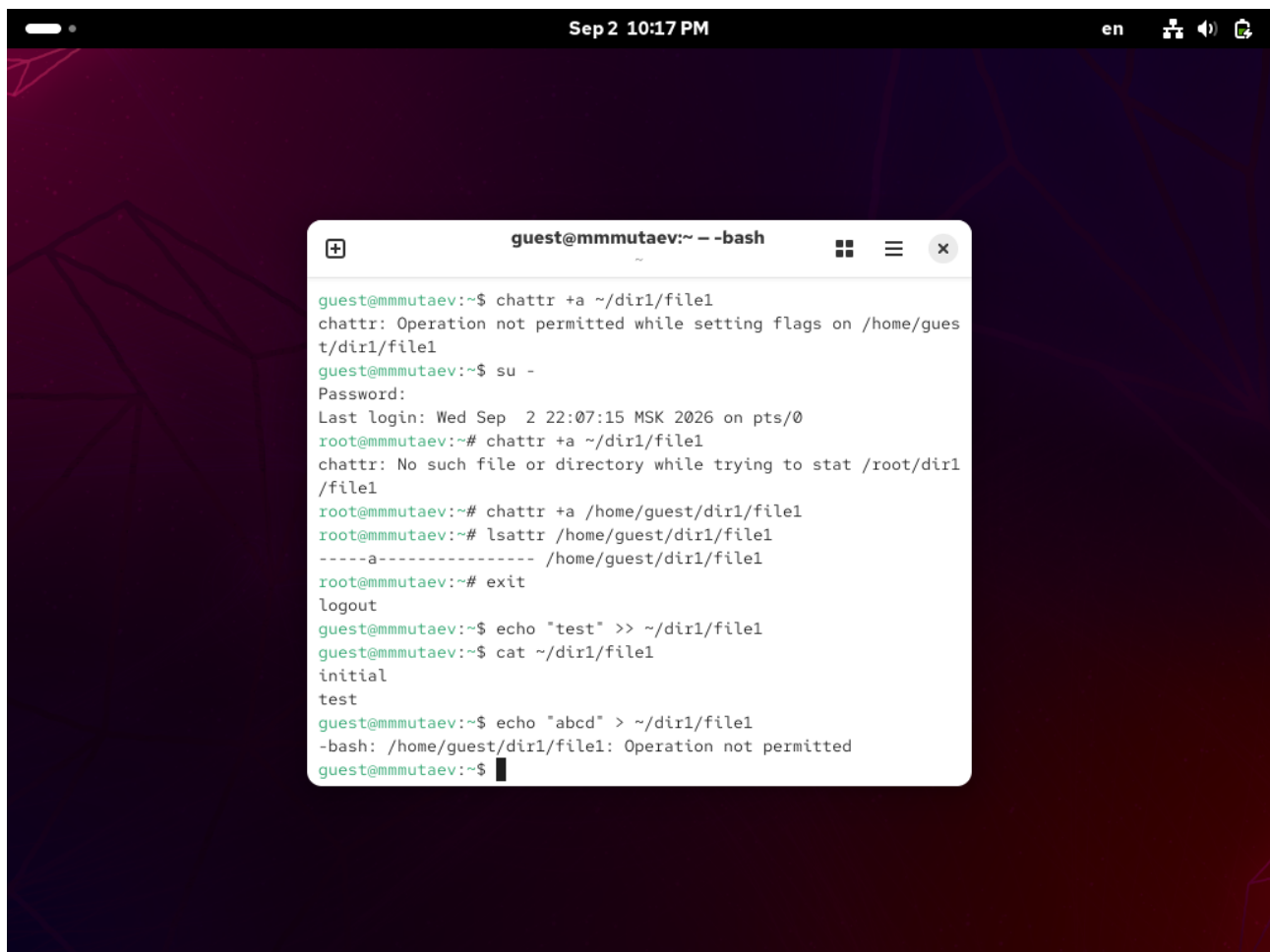
Рис. 4. Дозапись разрешена, перезапись запрещена.
