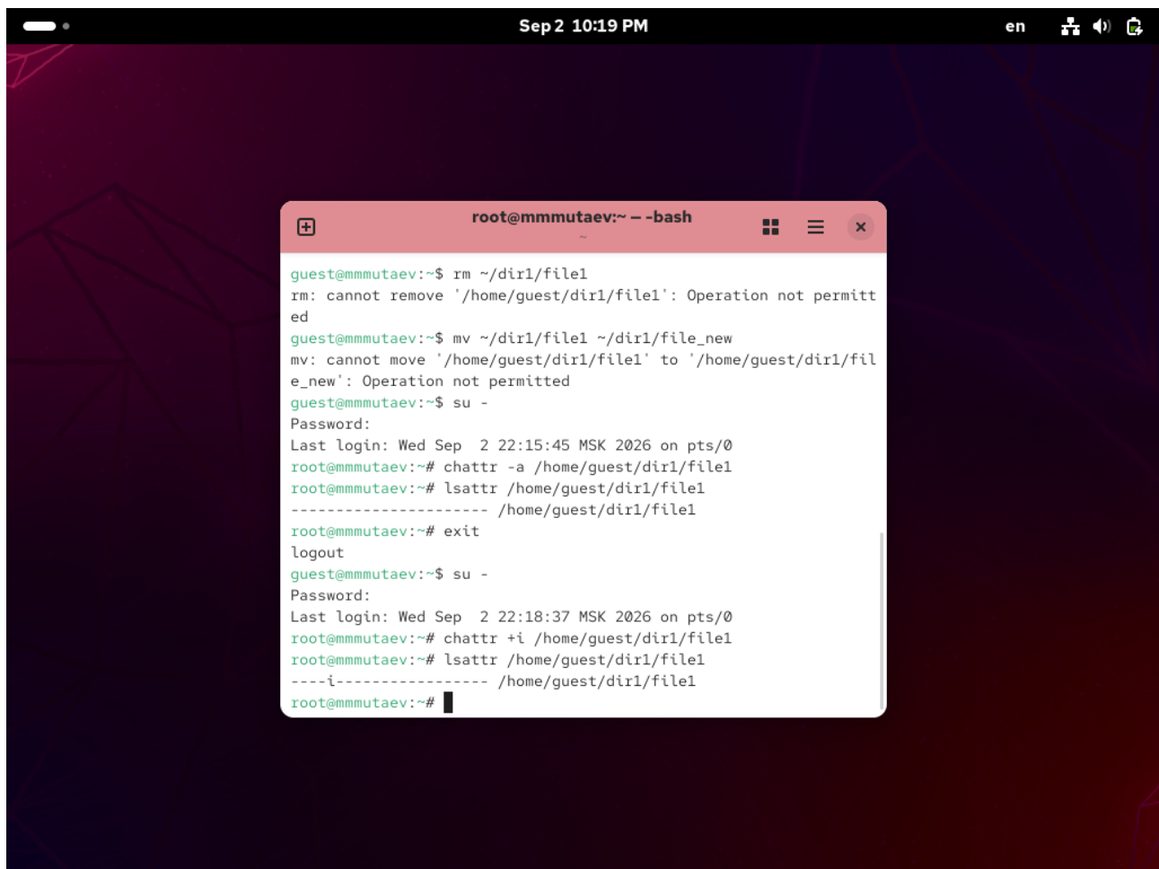
Рис. 7. Установка атрибута i.
