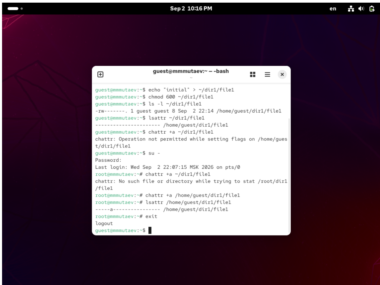
Рис. 3. Установка атрибута а.
