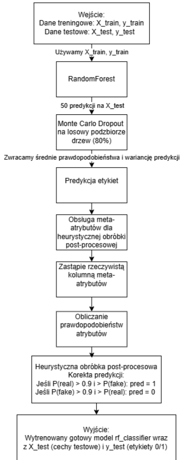
Rys. 2.10: Schemat metody 7.
