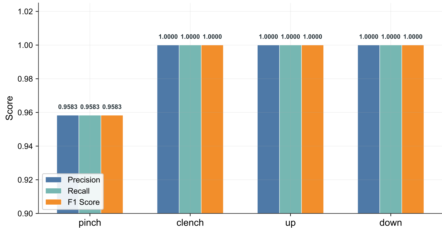
QEMU Validation: Per-Class Precision / Recall / F1
