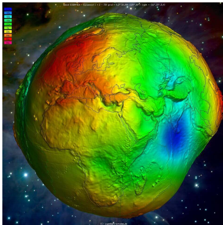
Figura 2.1: Raffigurazione del campo gravitazionale terrestre. Le differenze di esso fra le diverse regione del globo sono evidenziate tramite il colore e l'elevazione
