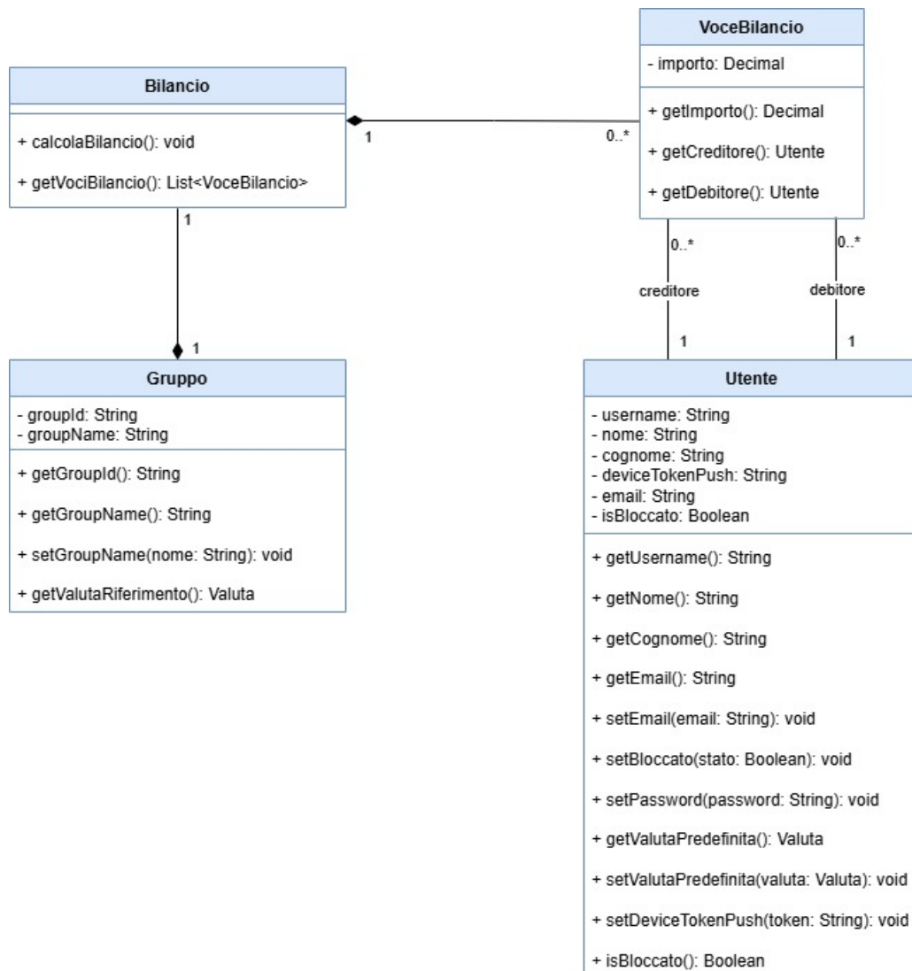
Figura 3.6: Modello del dominio: Bilancio in Progettazione
