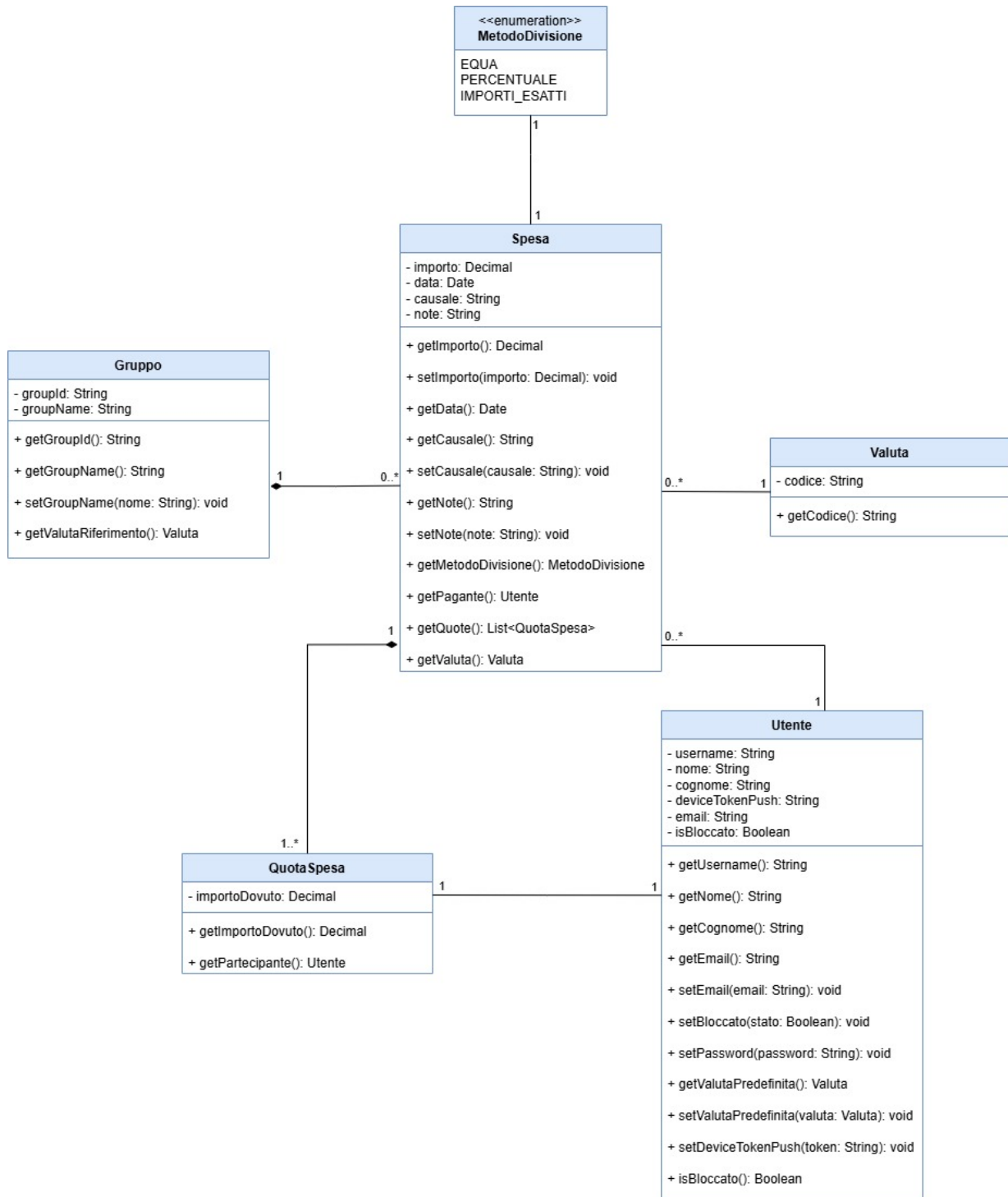
Figura 3.4: Modello del dominio: Spesa in Progettazione
