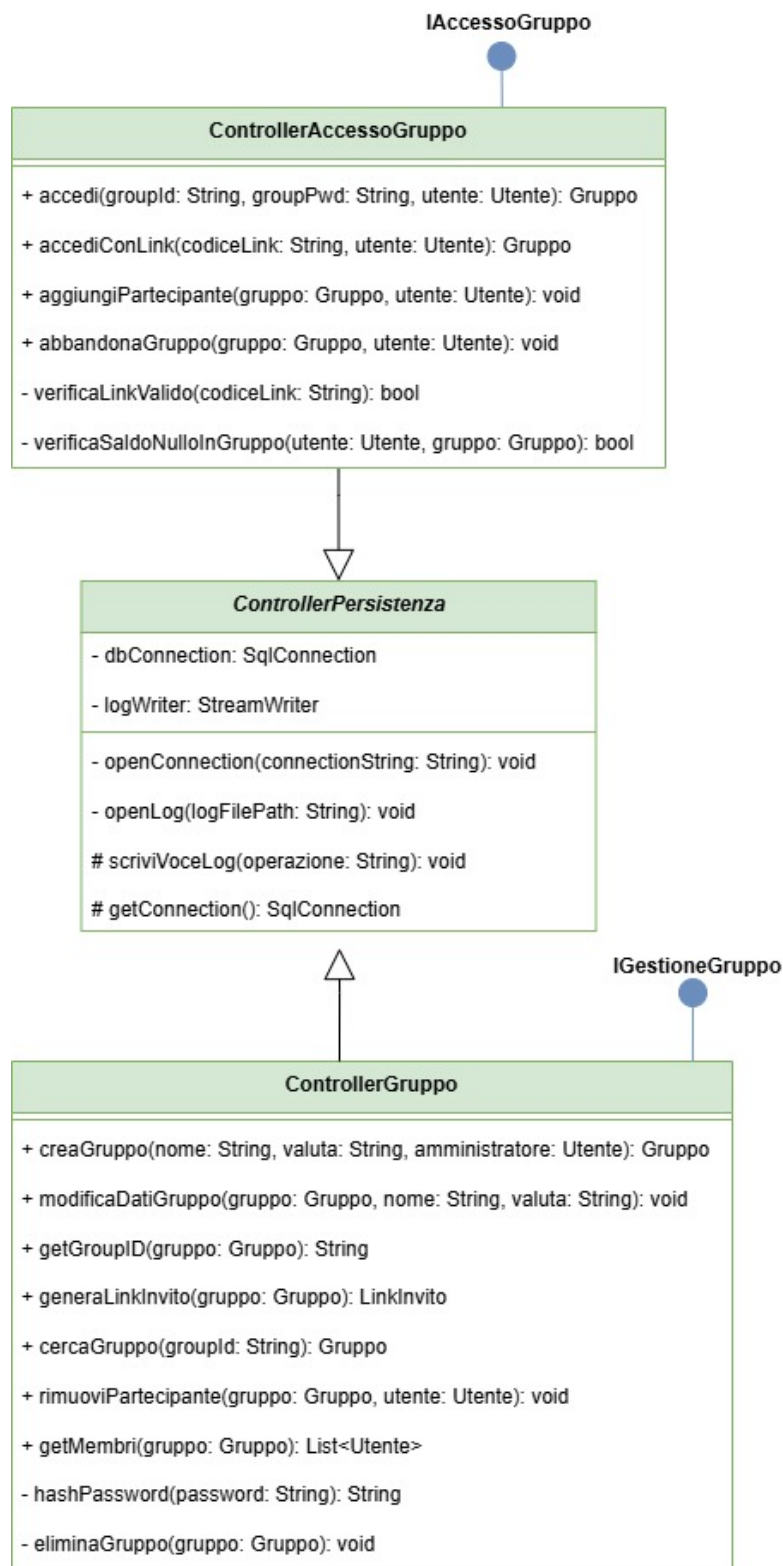
Figura 3.11: Controller: Accesso e Gestione Gruppo
