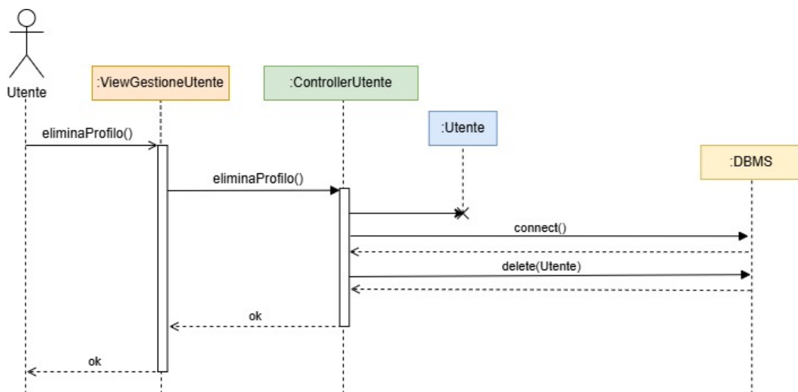
Figura 3.24: Diagramma di Sequenza: Elimina Profilo
