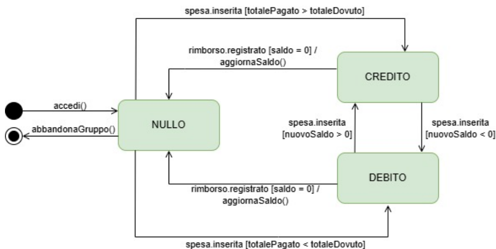
Figura 3.31: Diagramma di Stato: Saldo
