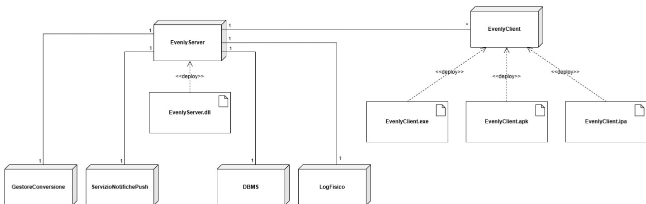
Figura 3.35: Diagramma di Deployment Type-Level
