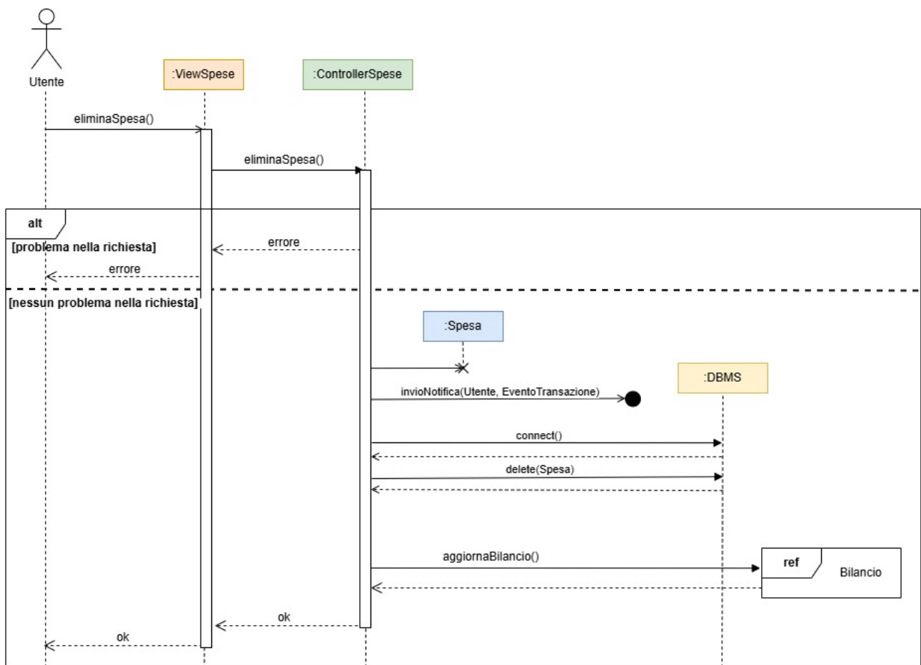
Figura 3.29: Diagramma di Sequenza: Elimina Spesa
