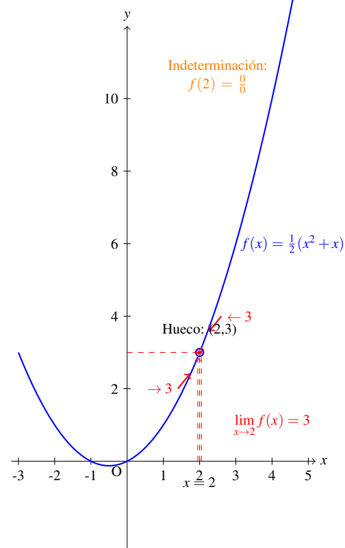
Figure 2: La función tiene una discontinuidad evitable en x = 2 . El límite existe y es 3, pero f(2) no está definida.
