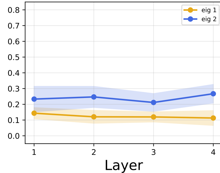
Wasserstein
