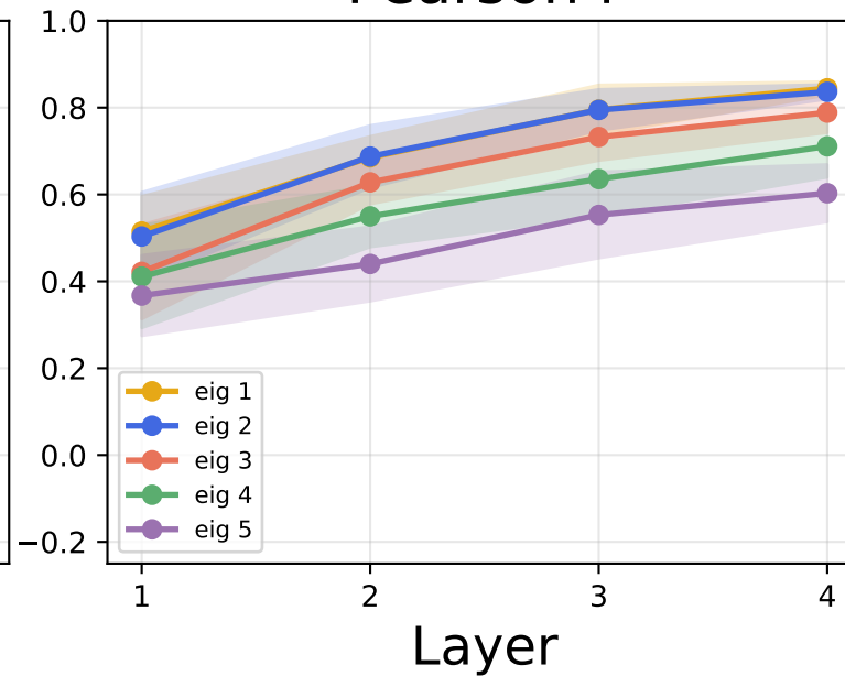
L2 raw
