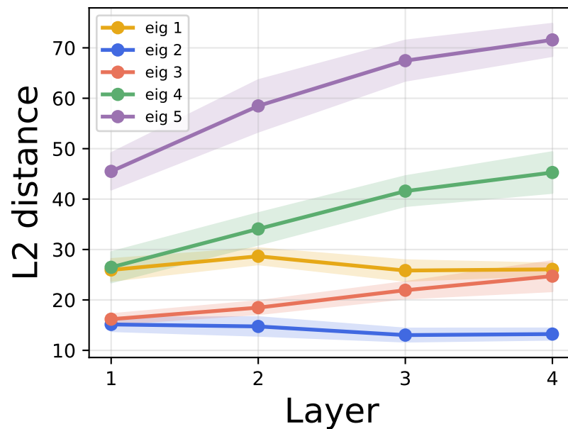
L2 raw
