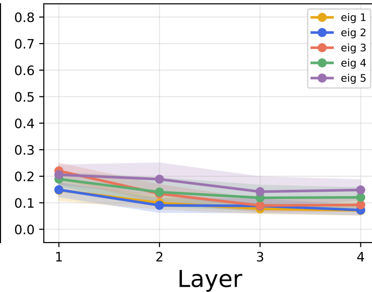
Wasserstein
