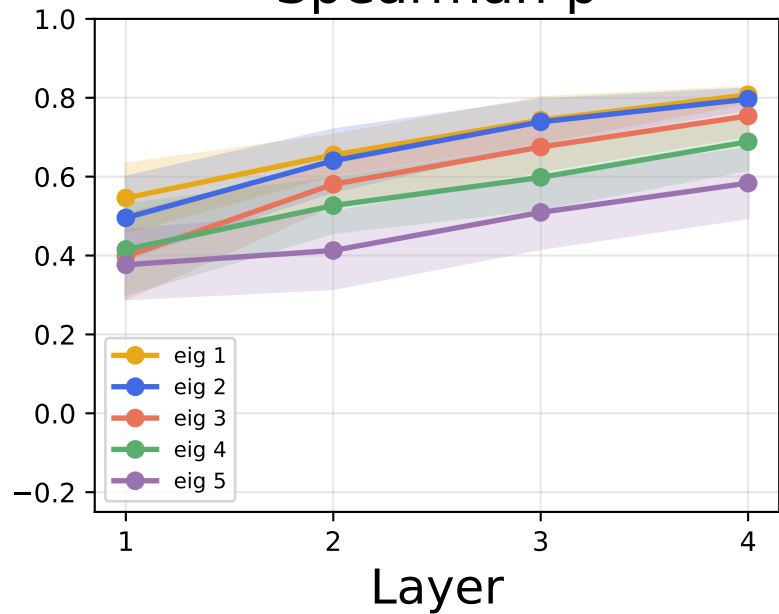
L2 raw
