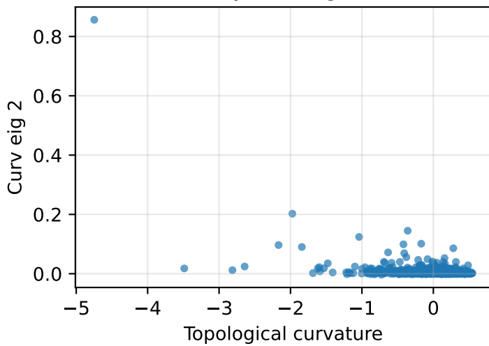
Layer 1, eig 2
