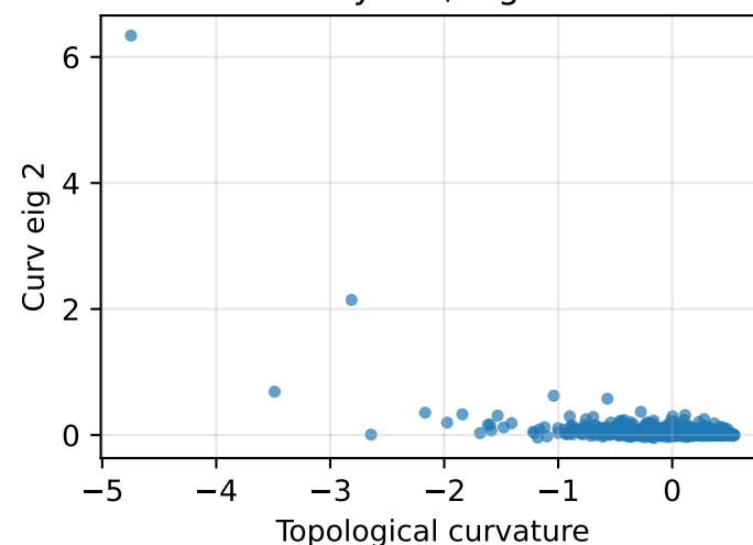
Layer 2, eig 2
