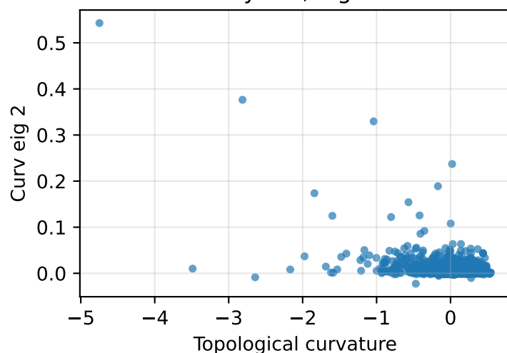
Layer 1, eig 2
