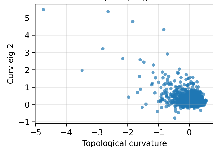
Layer 3, eig 2
