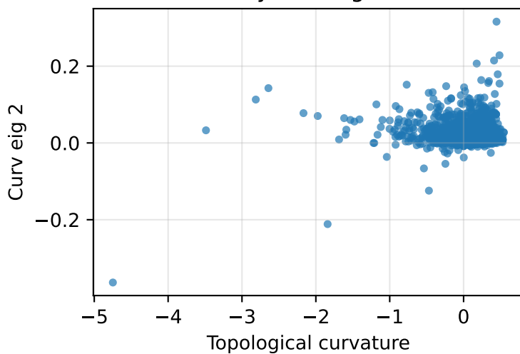
Layer 1, eig 2
