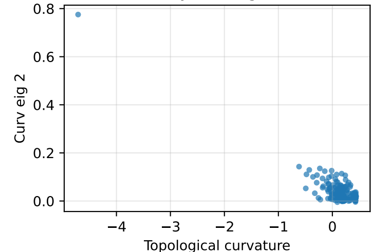
Layer 2, eig 2
