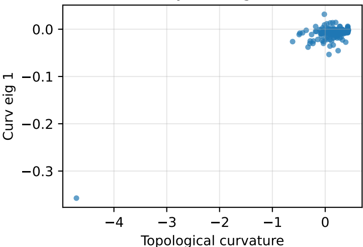
Layer 2, eig 1
