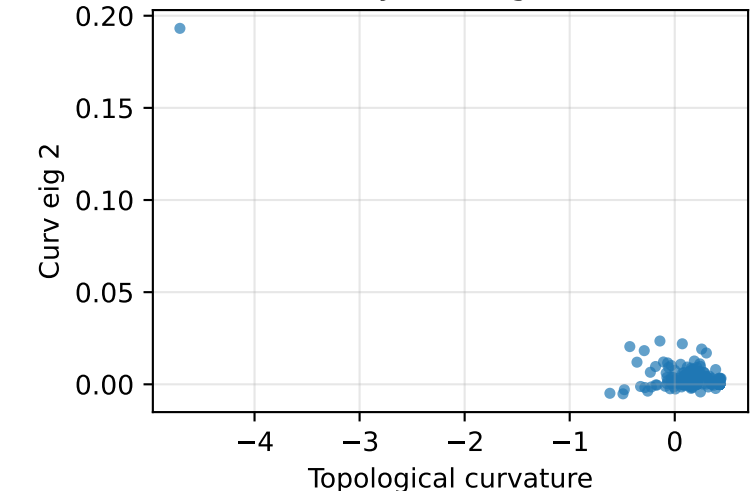
Layer 1, eig 2
