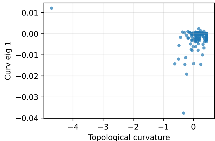
Layer 1, eig 1
