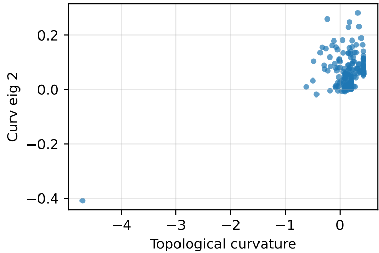
Layer 2, eig 2
