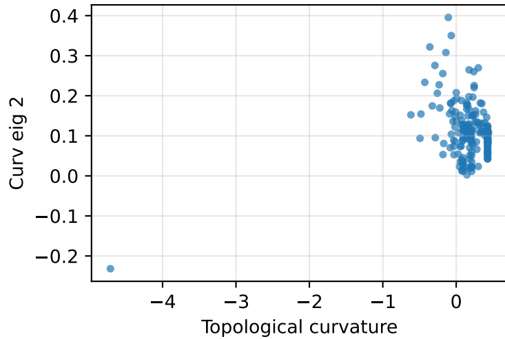
Layer 1, eig 2
