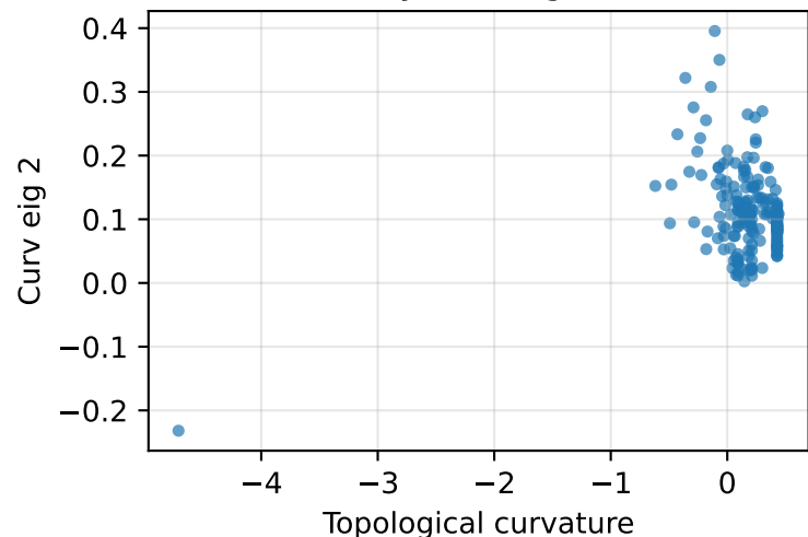
Layer 1, eig 2
