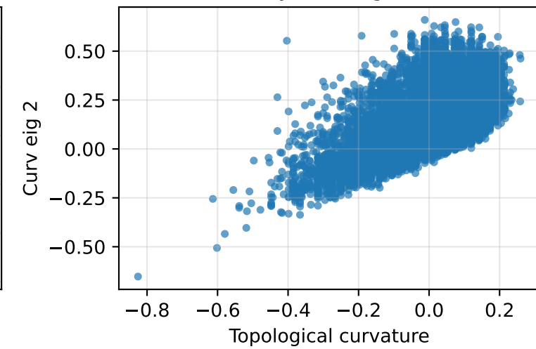
Layer 4, eig 2
