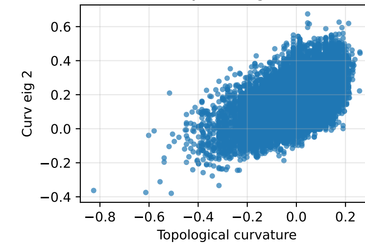
Layer 3, eig 2
