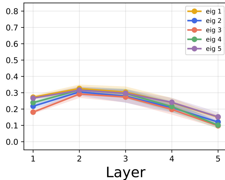
Wasserstein
