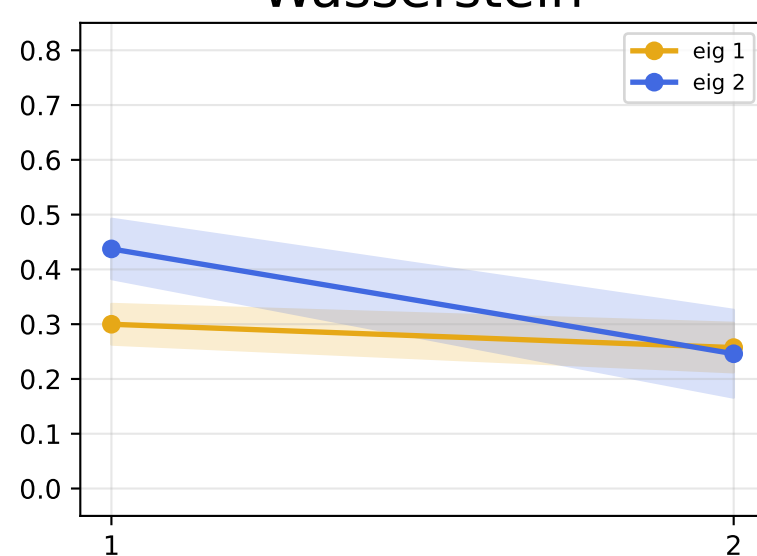
Wasserstein
