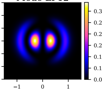
Mode LP12
