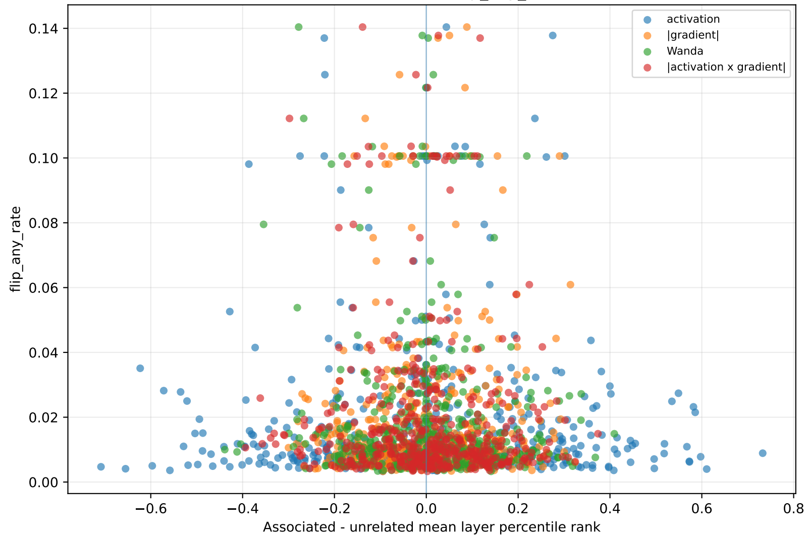
Metric contrast vs flip_any_rate
