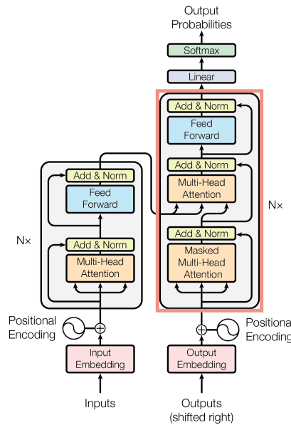
Figure 81: Struttura di un singolo blocco del decoder del Transformer con masked self-attention e cross-attention.
