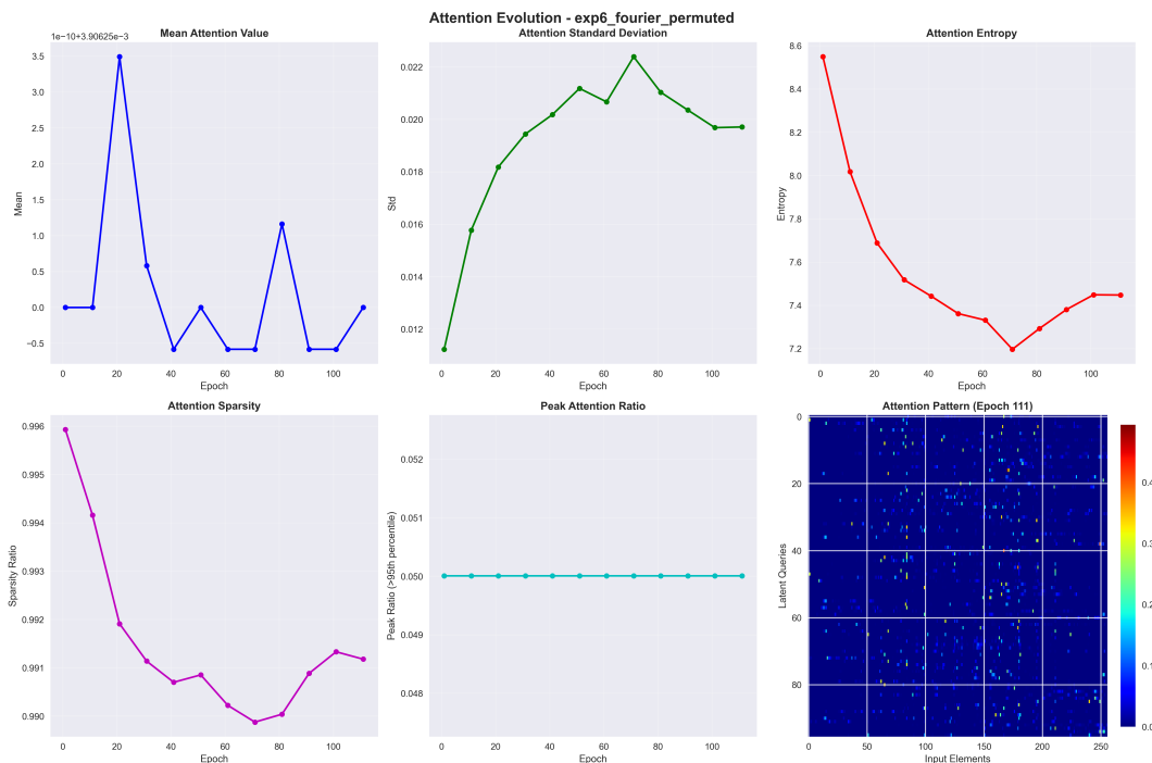
Figure 33: Evoluzione di exp6_fourier_permuted . Avvertenza: in questa run della prima generazione il flag --permute_pixels era definito ma mai letto dal codice, quindi i pixel non erano realmente permutati — la figura documenta la strutturazione dell’attention in condizioni normali, non sotto permutazione. La verifica quantitativa dell’invarianza è quella di e02_permuted nella §3.3, dove il flag è attivo e il calo (−2.68 punti) resta dentro la banda di rumore.
