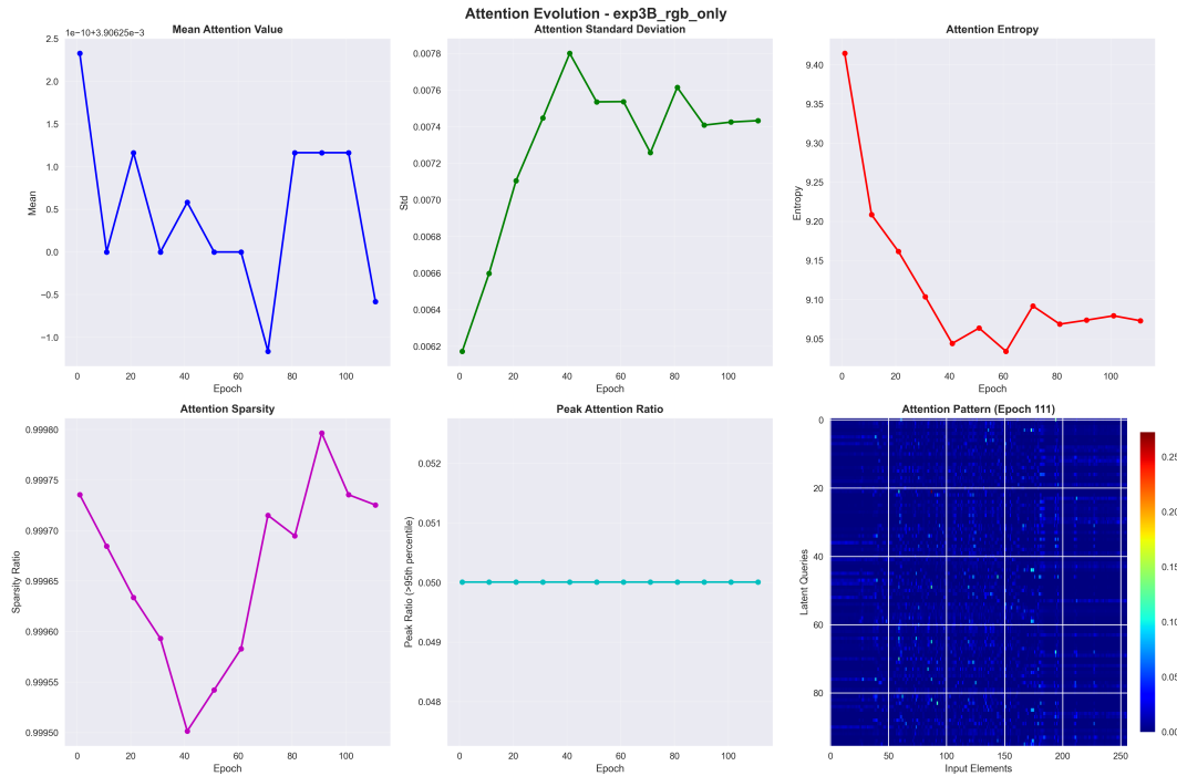
Figure 32: Evoluzione delle attention maps di exp3B_rgb_only (senza positional encoding). L'attention non si struttura nemmeno dopo molte epoche: entropia alta e costante ( \sim 9 ) — visivamente si vede che le teste continuano a guardare tutto l'input in modo quasi uniforme, confermando che senza PE il modello non può formarsi una “mappa” spaziale.
