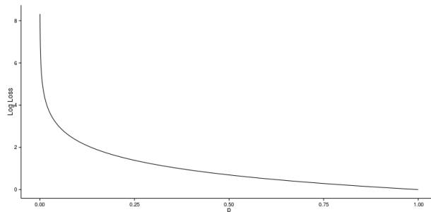
Figure 36: La funzione -\log(p) : quando la probabilità predetta p è vicina a 1, la loss è quasi zero; quando p \rightarrow 0 , la loss esplode verso +\infty . (Fonte: Wikimedia Commons)
