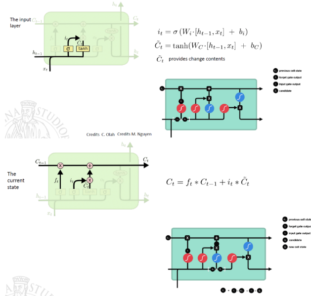
Figure 62: Sinistra: input gate e candidato ( i_t , \tilde{C}_t ). Destra: aggiornamento della cella di memoria ( C_t = f_t \odot C_{t-1} + i_t \odot \tilde{C}_t ).
