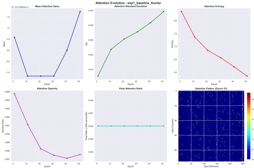
Figure 31: Evoluzione delle attention maps di exp1_baseline_fourier durante il training. All'epoca 1 l'attention è quasi uniforme; con il progredire del training emerge una struttura spaziale chiara, con i latenti che si specializzano su regioni diverse dell'immagine.
