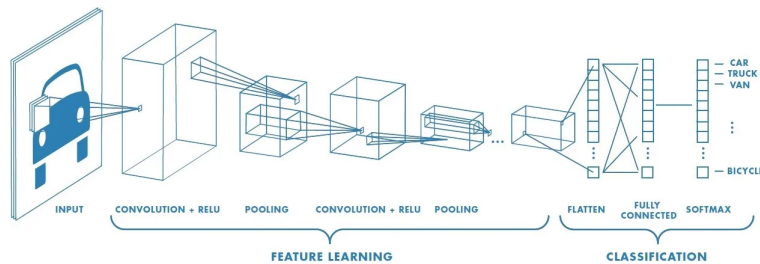
Figure 66: Architettura tipica di una CNN: convoluzioni, pooling e fully connected layer.
