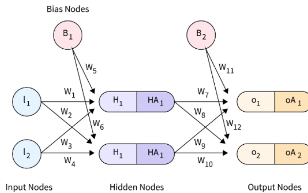
Figure 55: Architettura di una rete neurale feed-forward con input layer, hidden layer e output layer.
