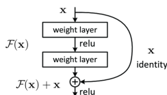
Figure 42: Il blocco residuale (da He et al., 2016): l'input \mathbf{x} attraversa due weight layer per calcolare F(\mathbf{x}) , poi viene sommato alla skip connection per ottenere F(\mathbf{x}) + \mathbf{x} .
