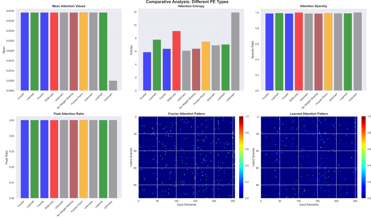
Figure 30: Analisi comparativa dei pattern di attention alla fine del training, per i 7 esperimenti CIFAR-10. Differenze nette tra Fourier PE (attention più strutturata, entropia \sim 6.4 ), Learned PE permuted (entropia \sim 7.8 , più diffusa), RGB-only (entropia \sim 9.1 , praticamente uniforme — il modello non sa dove guardare).
