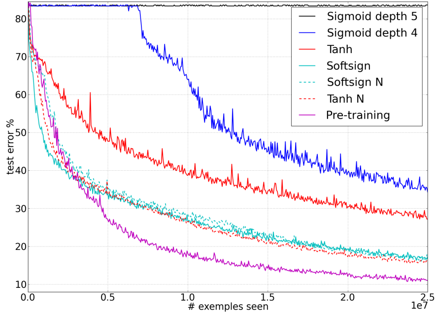
Figure 82: Test error per diverse attivazioni e inizializzazioni: l’inizializzazione normalizzata (Xavier/Glorot) raggiunge errori molto più bassi della sigmoide profonda che satura. Fonte: Glorot & Bengio (AISTATS 2010).
