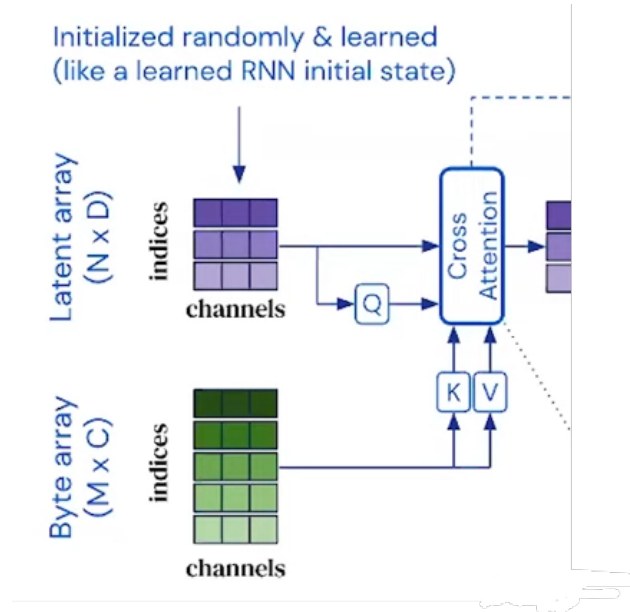
Figure 10: Schema complessivo della cross-attention: il latent array ( 512 \times 1024 ) proiettato a Q ( 512 \times 261 ) interroga il byte array ( 50\,176 \times 261 ) proiettato a K, V ( 50\,176 \times 261 ). Il prodotto QK^\top produce una matrice di attenzione rettangolare 512 \times 50\,176 .
