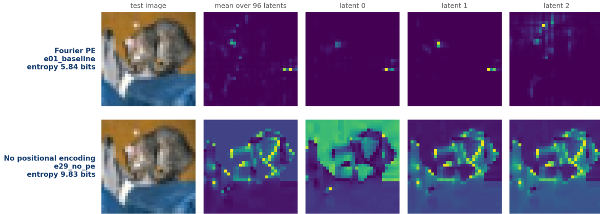
Figure 30: Cross-attention dell'ultimo stadio sulla stessa immagine di test. In alto e01_baseline (Fourier PE): latenti concentrati su pochi pixel, entropia media 5.84 bit. In basso e29_no_pe : attenzione che segue i confini di colore, 9.83 bit su un massimo di 10.
