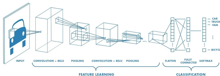
Figure 68: Architettura tipica di una CNN: convoluzioni, pooling e fully connected layer.
