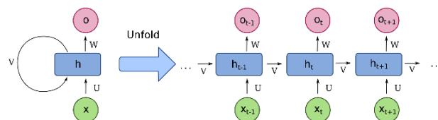
Figure 60: Schema di una RNN: il loop nello stato nascosto permette di mantenere memoria delle informazioni precedenti.
