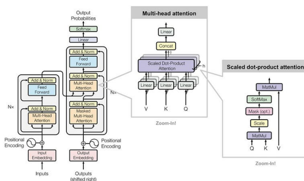
Figure 73: Architettura del Transformer: encoder (sinistra) e decoder (destra). Entrambi sono composti da blocchi ripetuti N\times contenenti attention + FFN + residual + LayerNorm.
