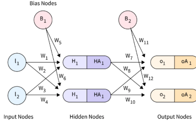
Figure 58: Architettura di una rete neurale feed-forward con input layer, hidden layer e output layer.
