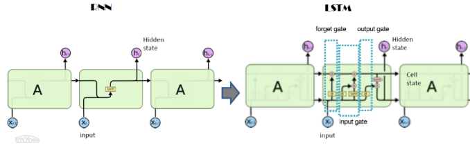
Figure 63: Struttura di una cella LSTM con le tre porte (forget, input, output) e la cella di memoria.
