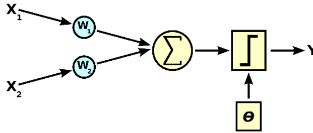
Figure 55: Struttura di un neurone artificiale: input x_i , pesi w_i , somma ponderata e funzione di attivazione.
