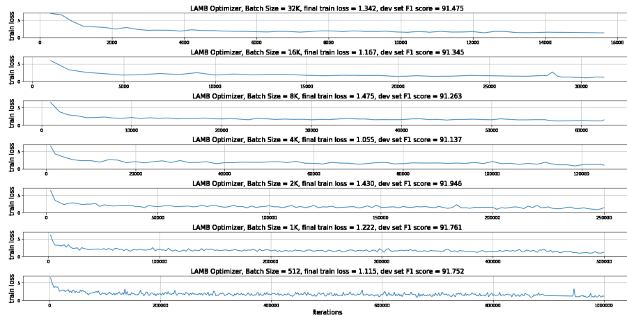
Figure 47: Training di BERT con l'ottimizzatore LAMB a batch crescenti (512–32K): la qualità finale (F1 \approx 91.5) si mantiene anche con batch enormi — è l'optimizer usato nel nostro progetto. Fonte: You et al., LAMB (arXiv:1904.00962).
