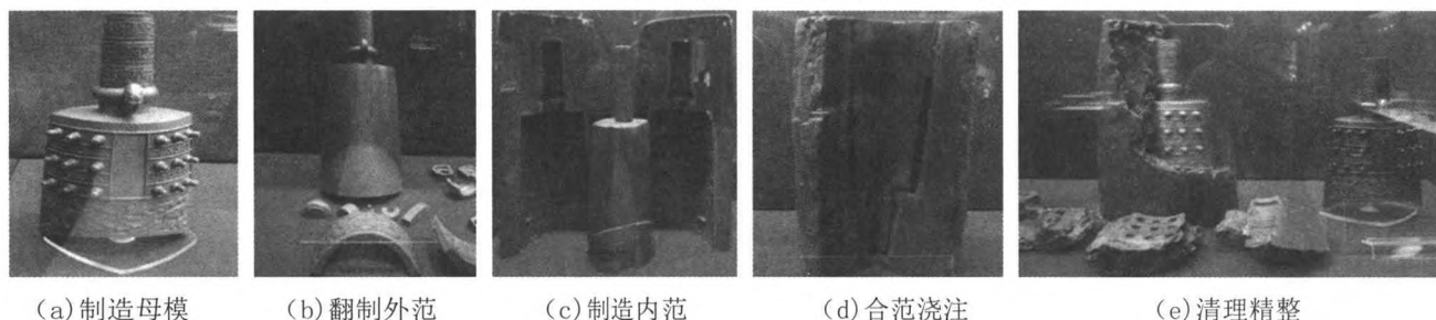
图 4 传统泥范铸造流程 (上海博物馆)
