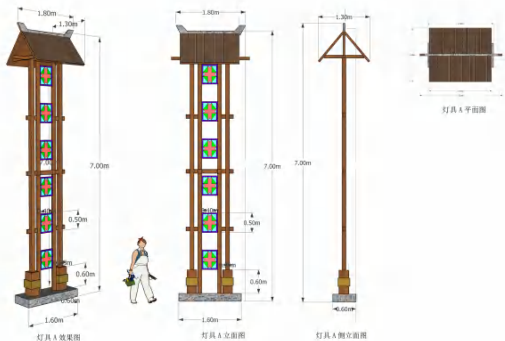
图 4.33 灯具 A 设计图
