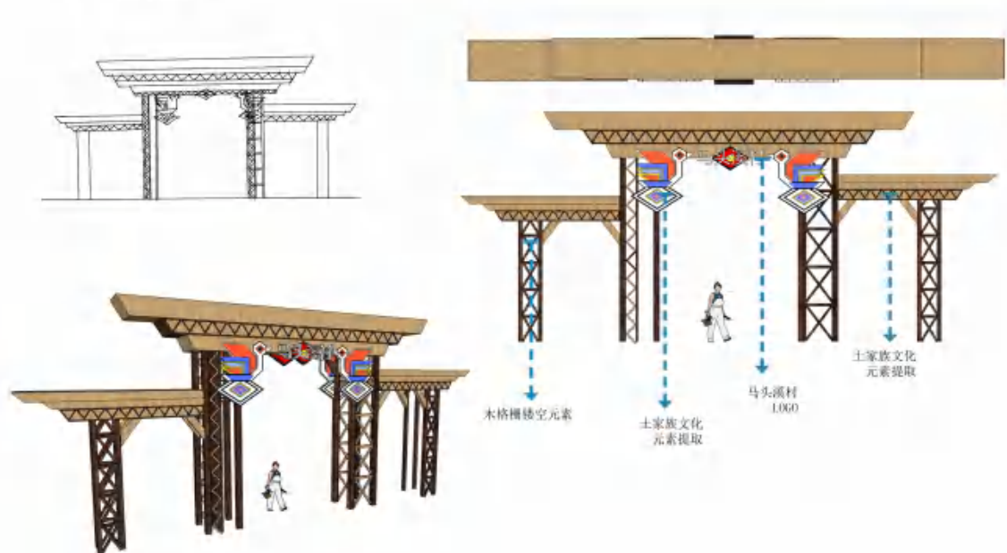
图 4.30 寨门小品设计图
