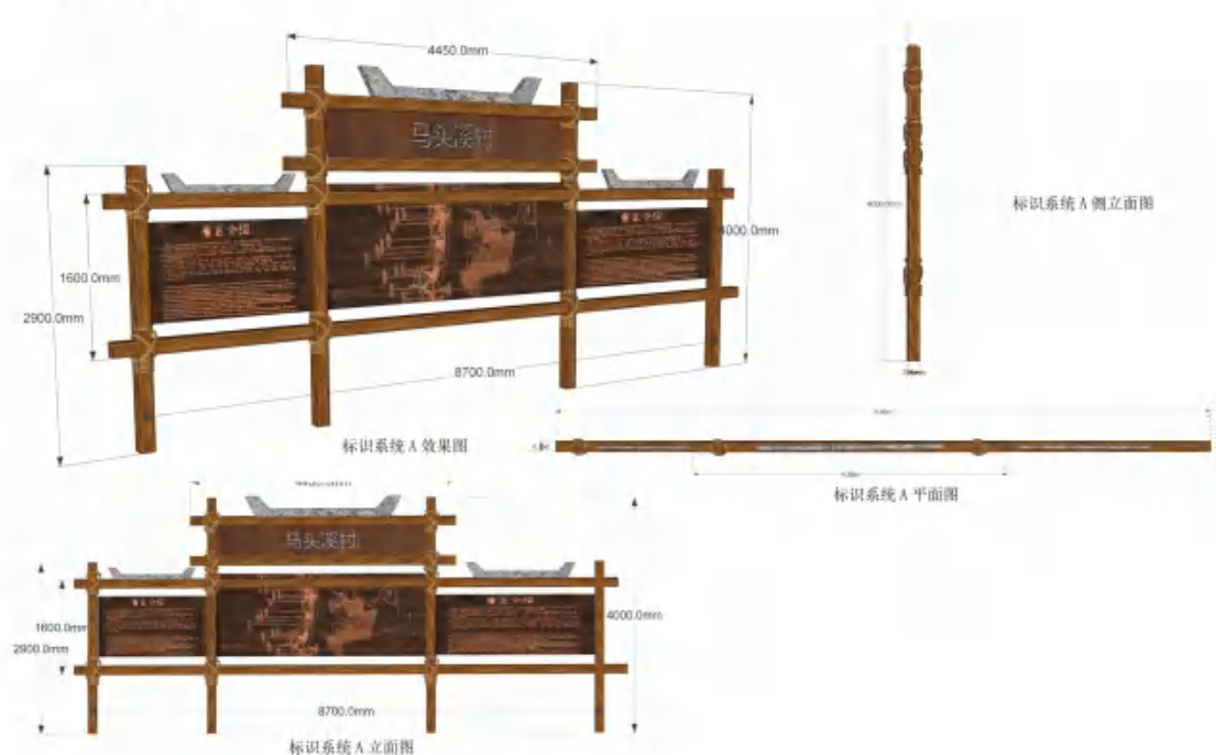
图 4.31 标识系统 A 设计图
