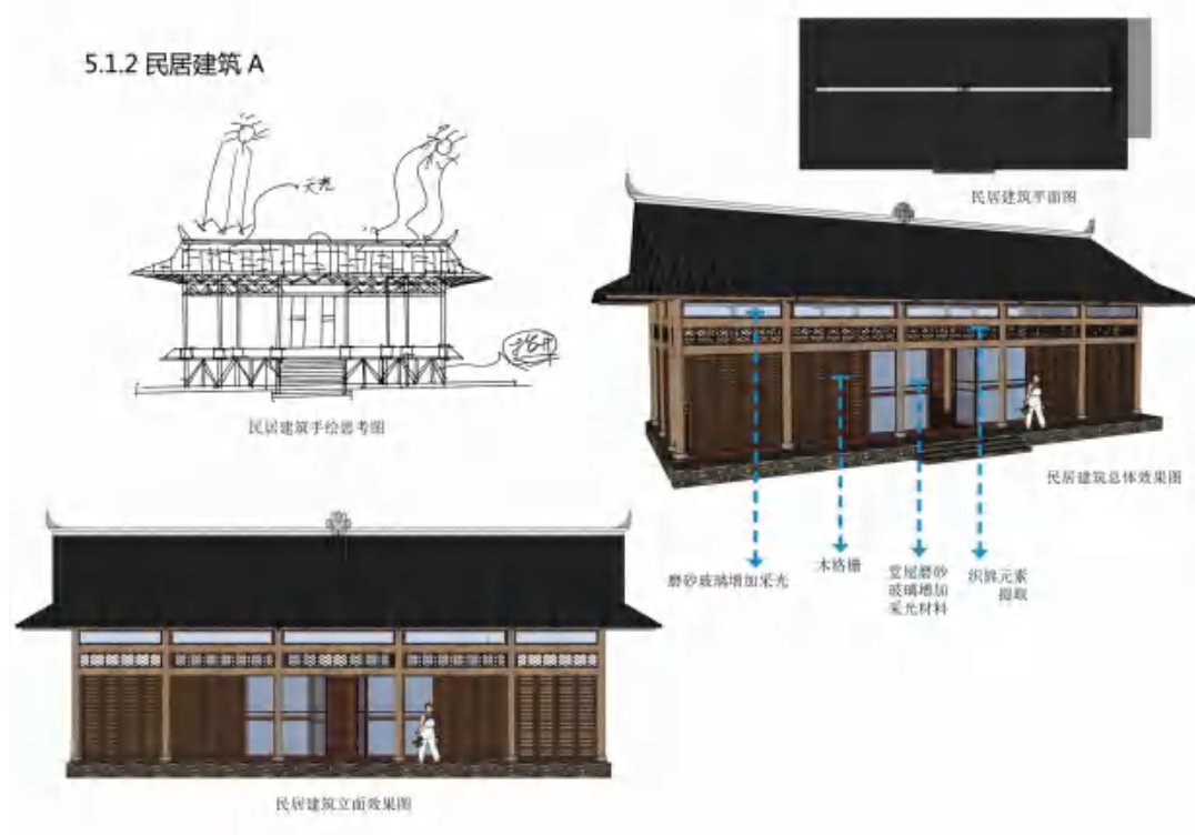
图 4.36 民居建筑 A 设计图
