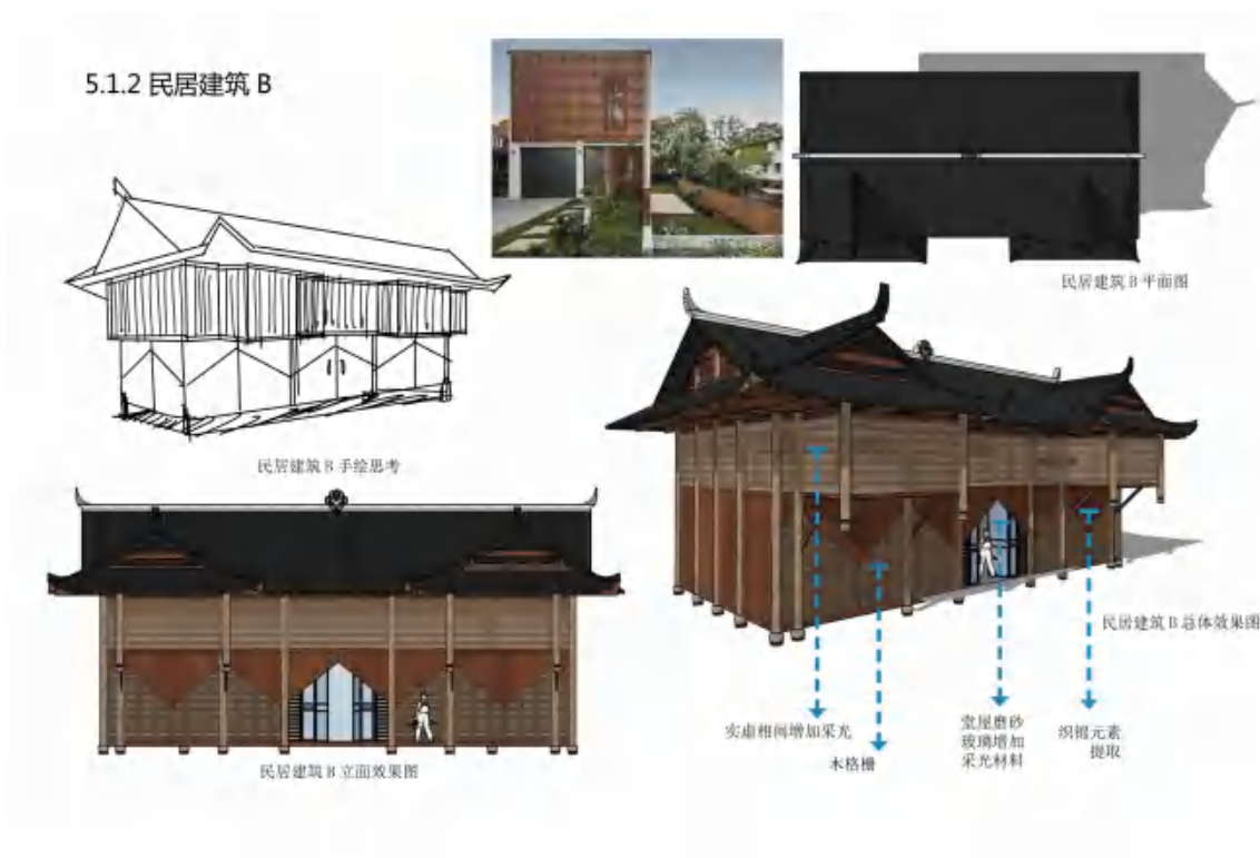
图 4.37 民居建筑 B 设计图
